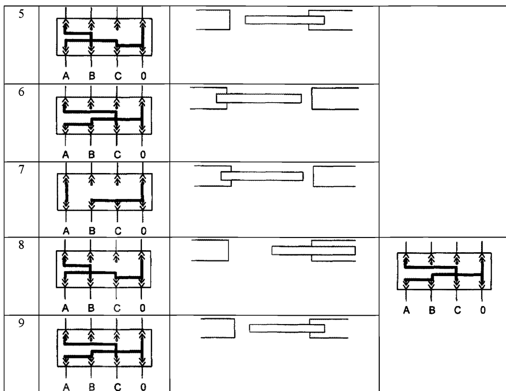
Рис. 27. Проверка правильности фазировки цепей тока по концам ВЛ:
