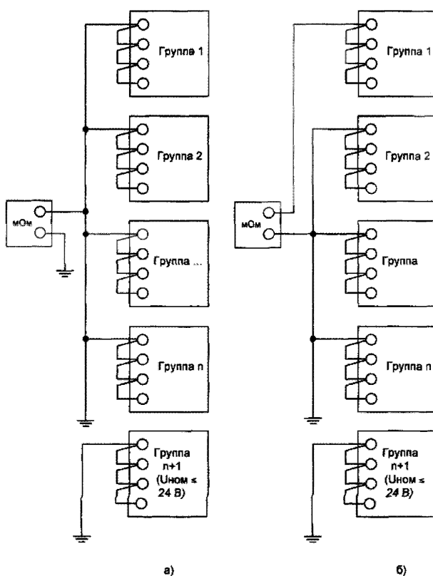
Рис. 3. Схема измерения сопротивления изоляции:
