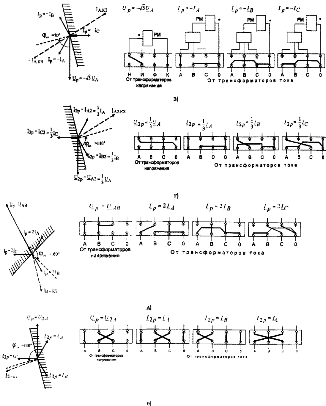
Рис. 21. Определение ожидаемого поведения реле мощности при подведении рабочих токов и напряжений:
