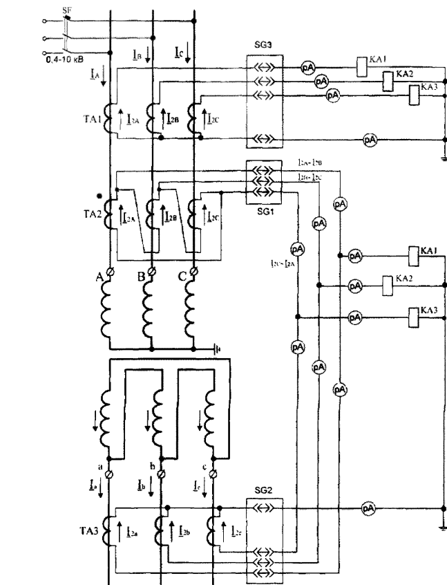
Рис. 13. Схема проверки защит трансформатора первичным током от трехфазного источника
