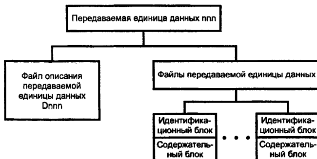
Рисунок 2 — Логическая структура передаваемой единицы данных
