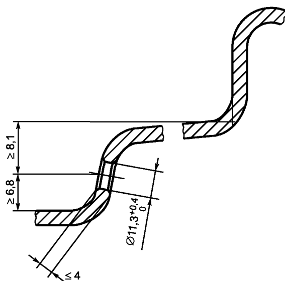
Рисунок 3 — Размеры вентиляного отверстия для бескамерных шин
