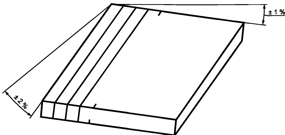
Рисунок 2 — Характеристики лотков
