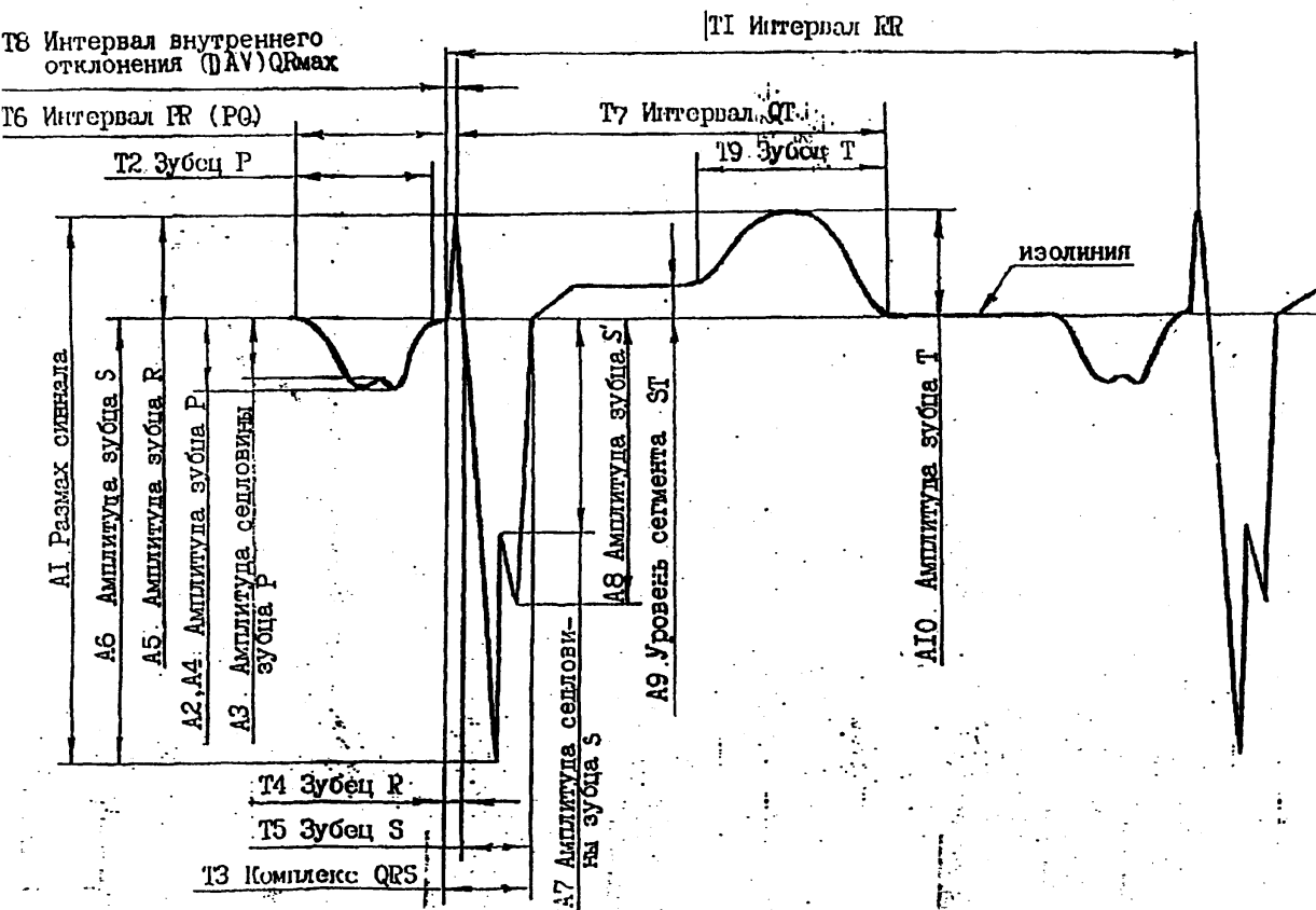
Рисунок А.3 – Наименования амплитудно-временных параметров элементов испытательного ЭКГ-
