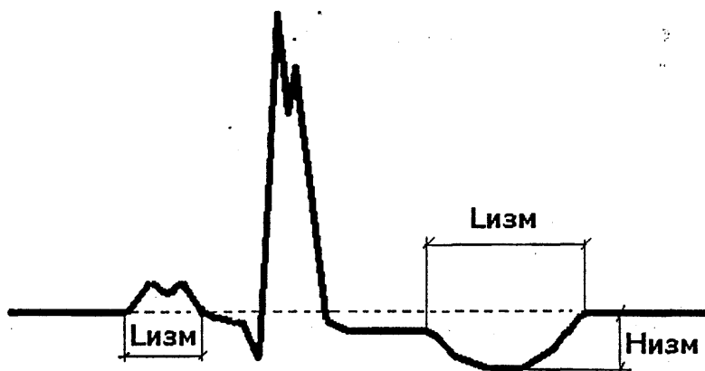
Рисунок 3 - Обозначения фрагментов тестового ЭКГ-сигнала
