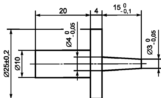
Рисунок 2 — Испытательный щуп
