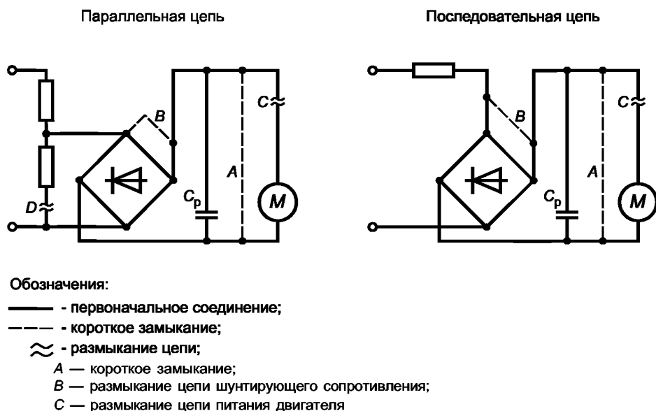
Рисунок В.1 — Схема имитации неисправностей
