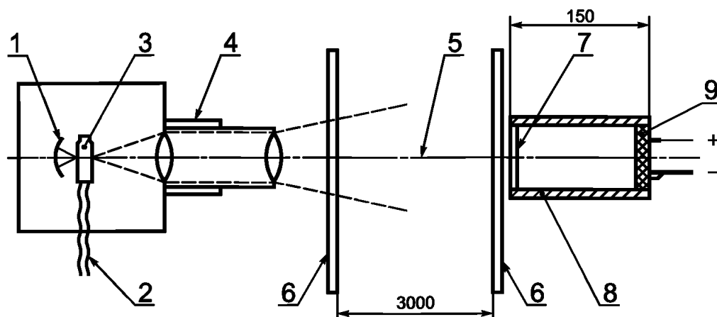
Рисунок 1 — Схема плана испытательной камеры (вид сверху)
