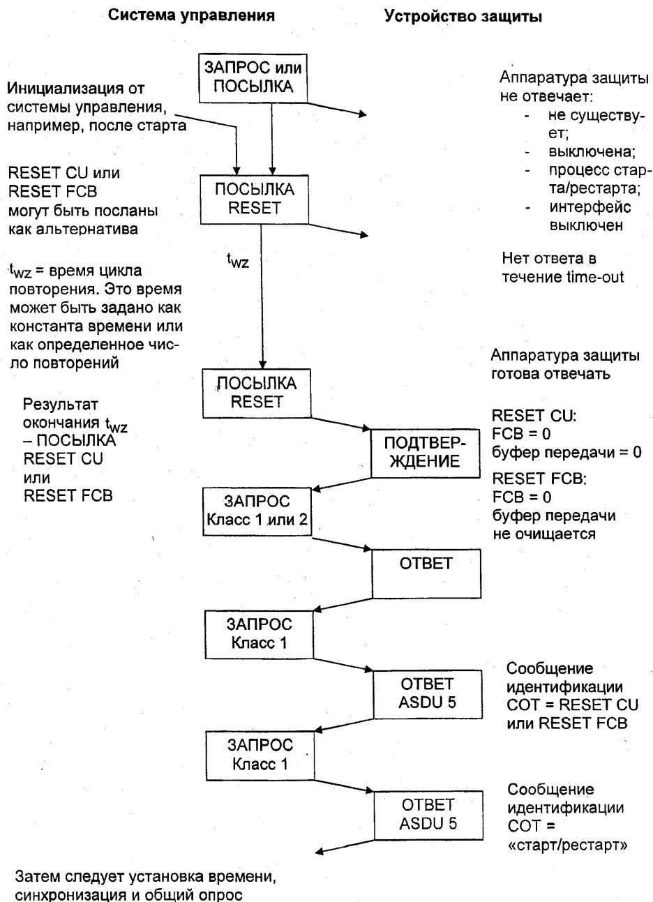
Рисунок 3 — Основная процедура инициализации
