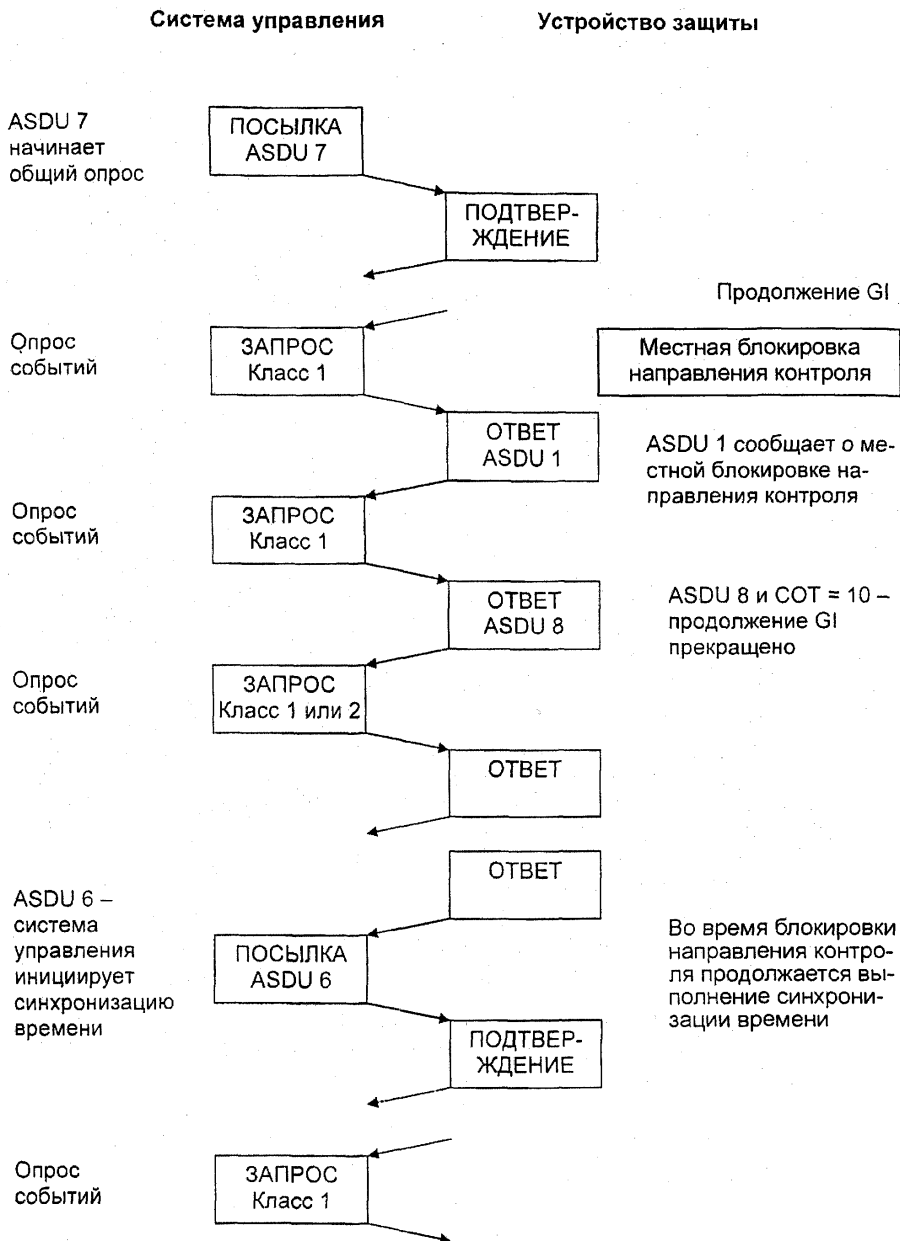
Рисунок 9 — Блокировка направления контроля (лист 1)
