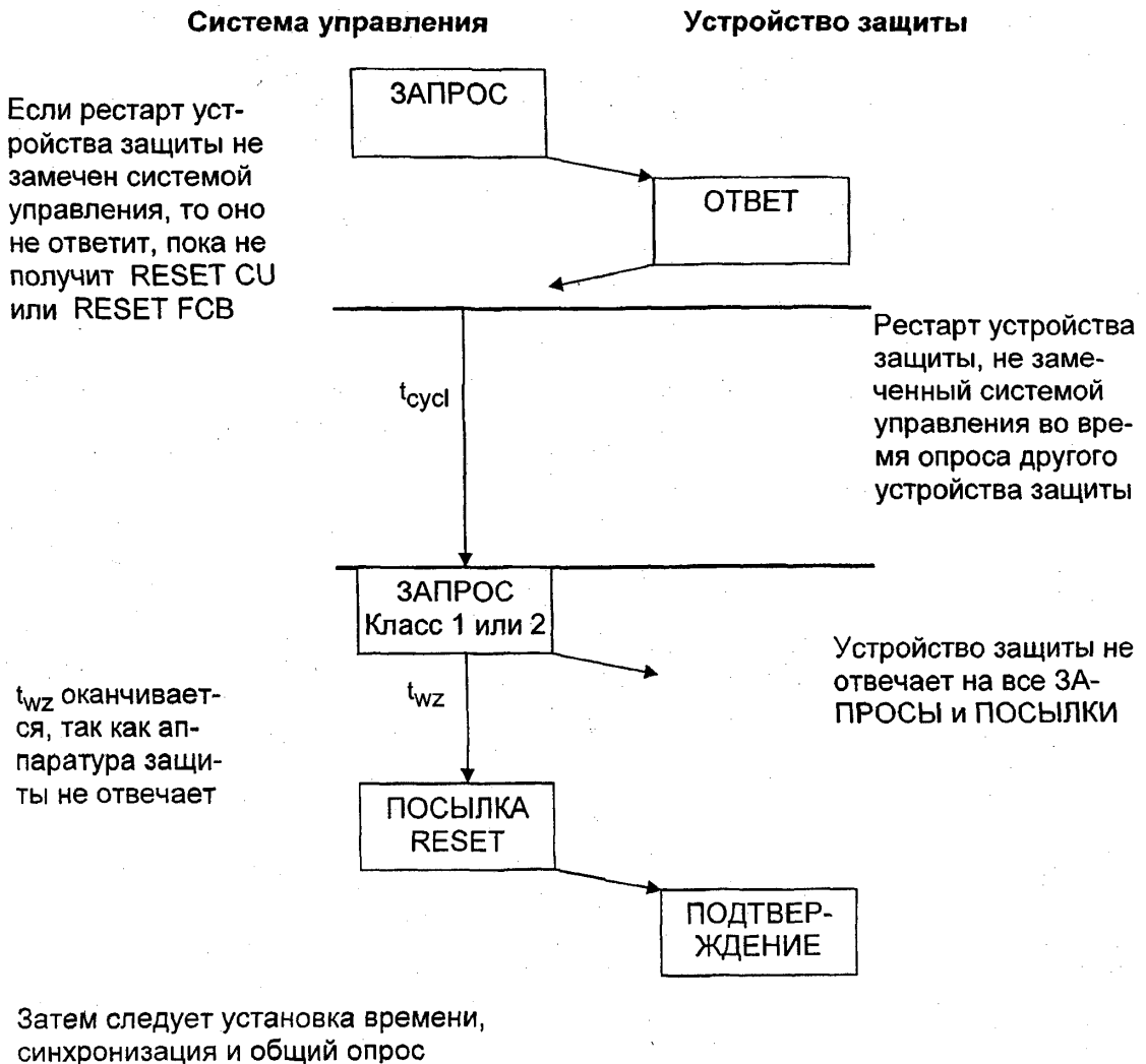
Рисунок 4 — Процедура инициализации после рестарта аппаратуры защиты
