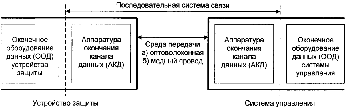
Рисунок 1 — Интерфейсы и соединения между устройством защиты и системой управления
