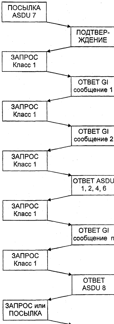
Рисунок 6 — Общий опрос
