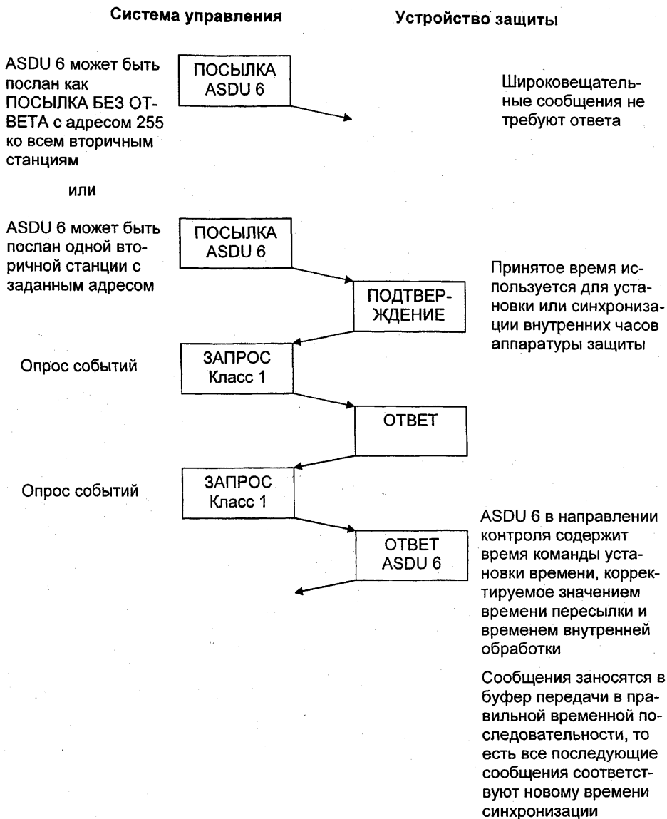
Рисунок 5 — Синхронизация времени
