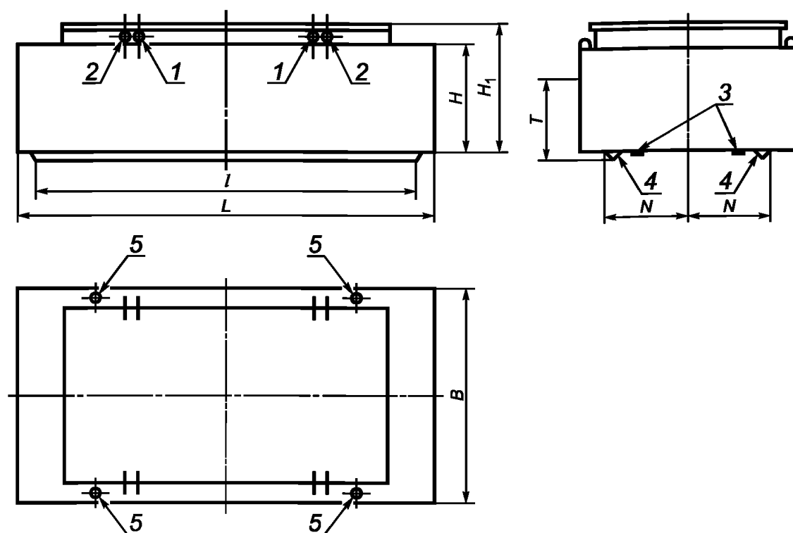
1 — места присоединения пожарных шлангов; 2 — места присоединения шлангов подачи \text{CO}_2 ; 3 — накладные листы под домкраты; 4 — направляющий угольник размерами 150 \times 150 \times 12 мм; 5 — установочные тумбы
