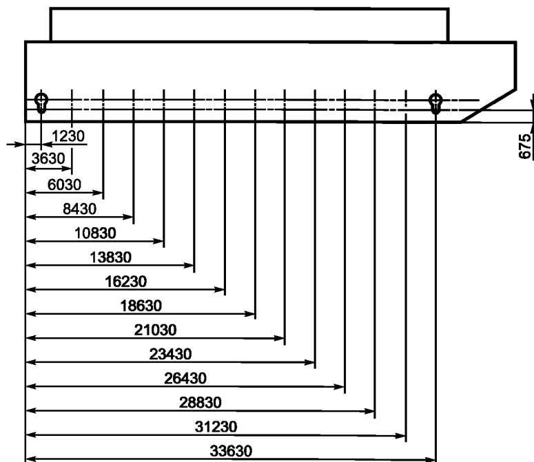
Рисунок 2 — Расположение бортовых гнезд
