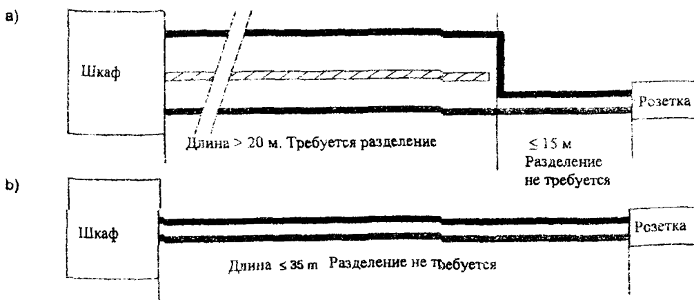
Рис. 18. Разделение силовых и информационных кабелей
