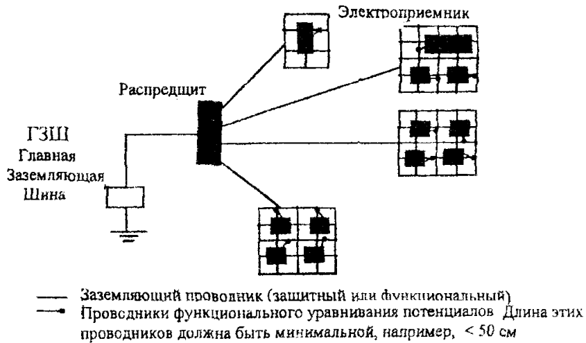
Рис. 14. Пример радиально-сетчатой системы уравнивания потенциалов (Основа – радиальная сеть. На конце каждого радиуса – местное сетчатое уравнивание.)
