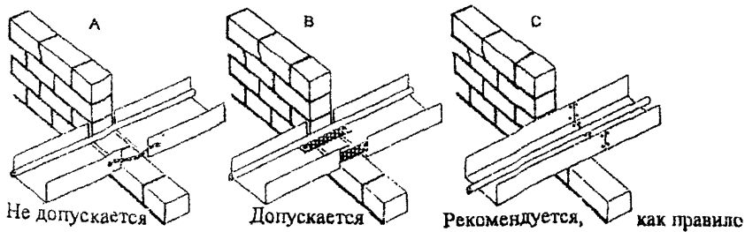
Рис. 25. Соединение секций металлических лотков в местах прохода сквозь стену
