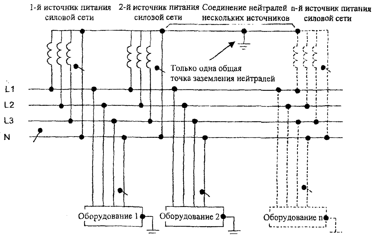
Рис. 8. Питание от нескольких источников в системе TT с заземлением нейтралей источников в одной общей точке
