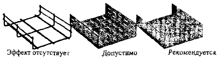
Рис. 21. Влияние конструкции металлических лотков на уровень электромагнитной совместимости
