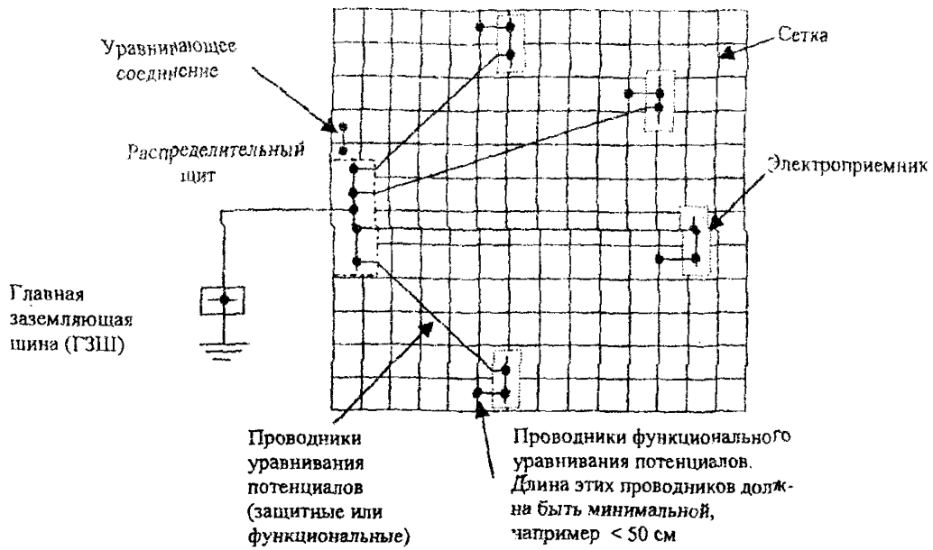
Рис. 15. Пример сетчато- радиальной системы уравнивания потенциалов (Основа – сетчатая структура большой площади, на которой размещена радиальная сеть)
