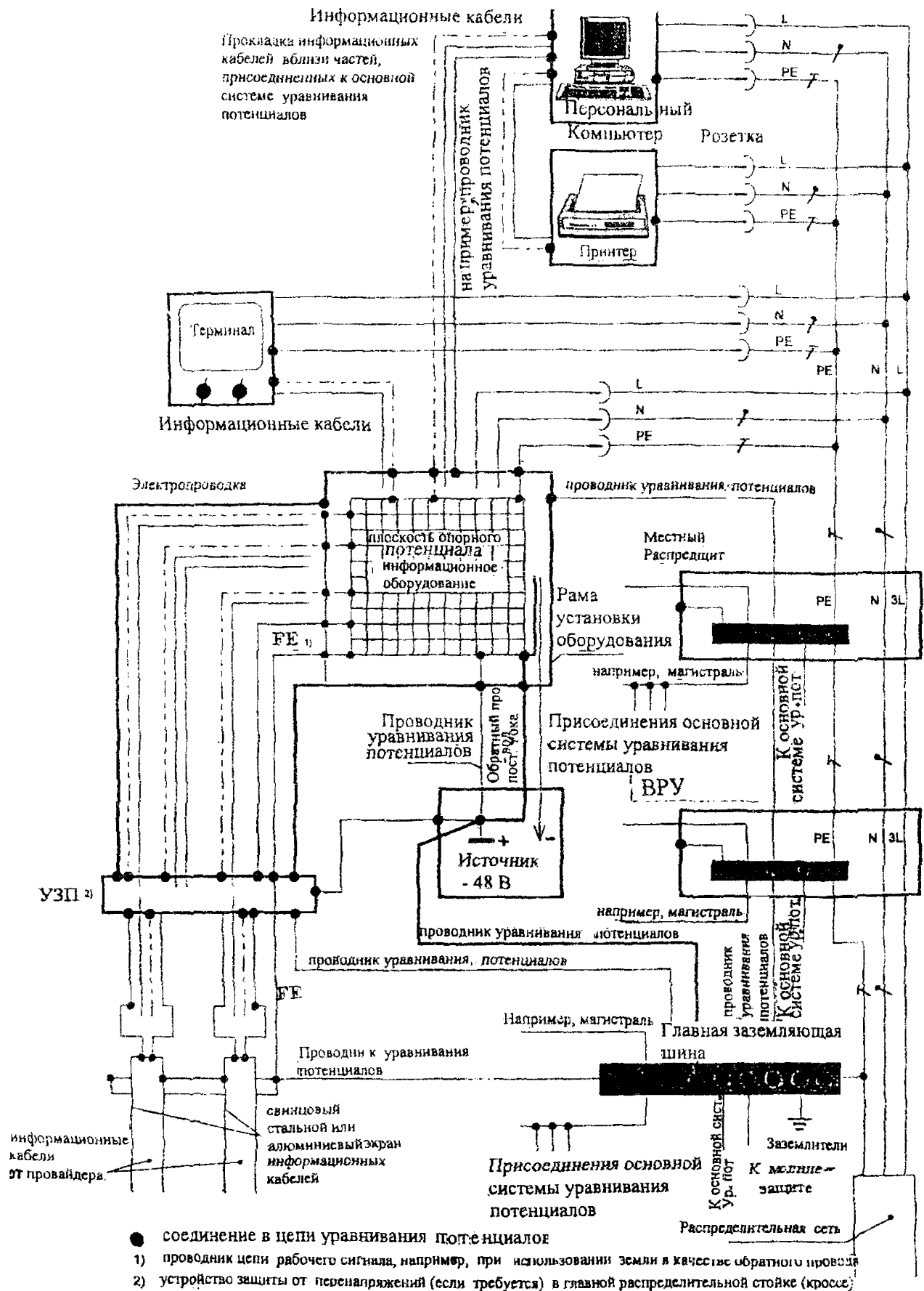
Рис. 11 Д. Пример улучшенной (сложной) системы уравнивания потенциалов информационного оборудования в здании
