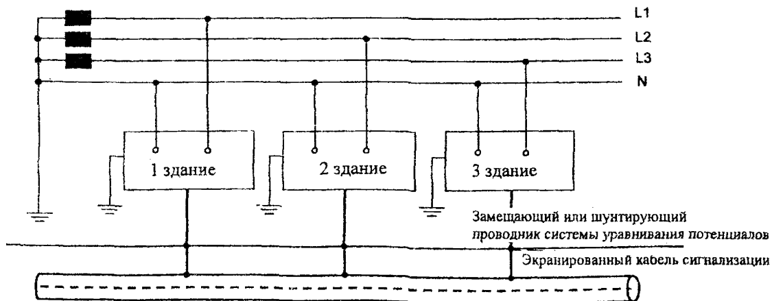
Рис. 2. Пример замещающего или шунтирующего проводника уравнивания потенциалов в системе ТТ
