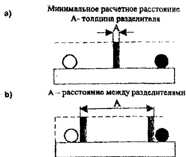
Рис. 19 В . Пример параллельной прокладки силовых и информационных кабелей, разделенных перегородкой (разделителем).
