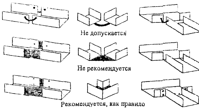
Рис. 23. Соединение секций металлических лотков
