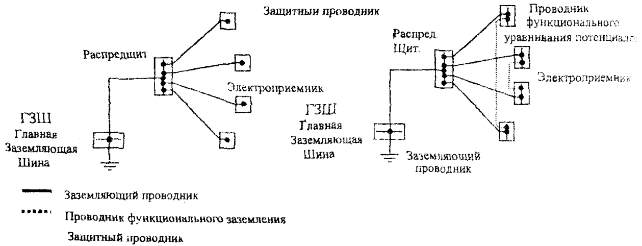
Рис. 13. Пример радиального соединения защитных проводников ( звезда)
