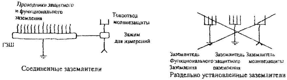
Рис. 12. Соединение заземлителей
