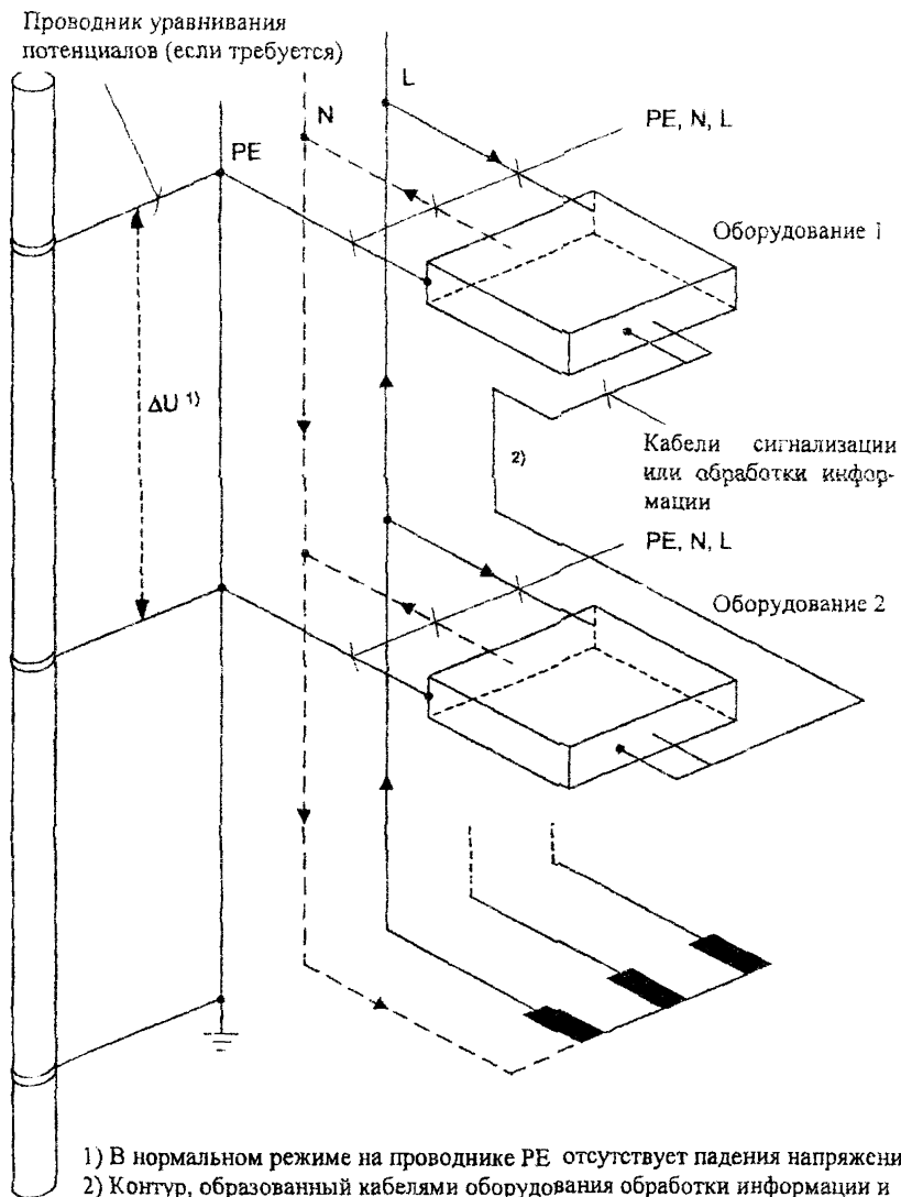
Рис. 6. Система IT в электроустановке здания
