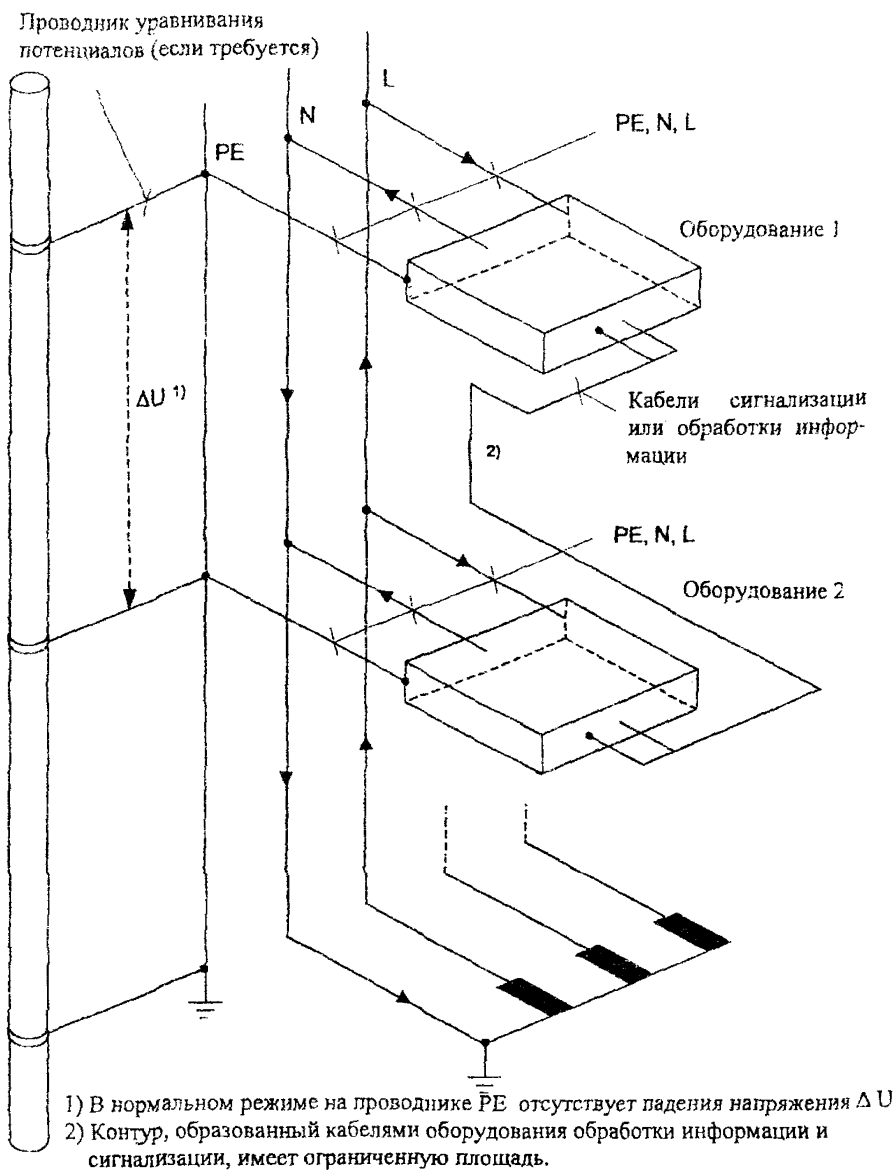
Рис. 5. Система ТТ в электроустановке здания.
