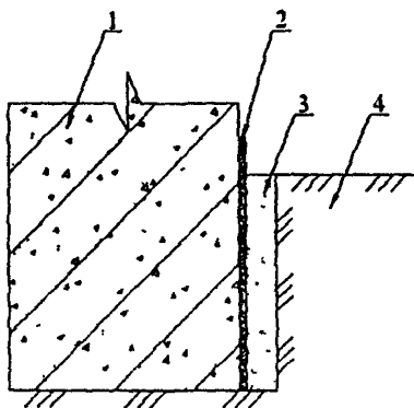
Рис. 17. Внешняя герметизация и утепление заглубленных конструкций
