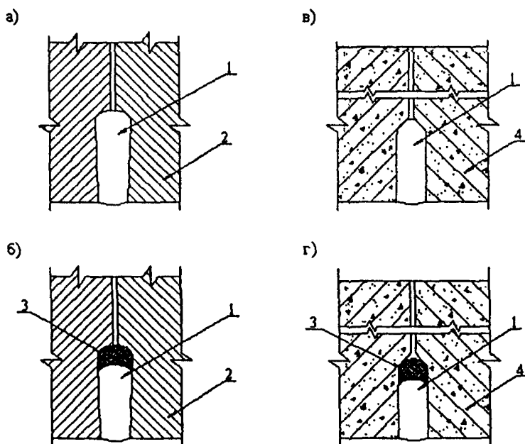
Рис. 21. Гидроизоляция стыков чугунной (а, б) и сборной железобетонной отделки (в, г) закрытого способа работ:
