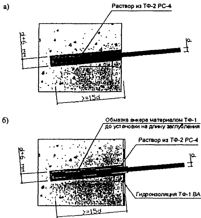
Рис. 8. Закрепление анкера
