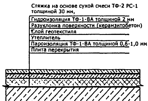
Рис. 9. Устройство кровли
