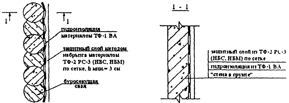
Рис. 6. Устройство гидроизоляции и защитного слоя «стены в грунте», буросекущие сваи
