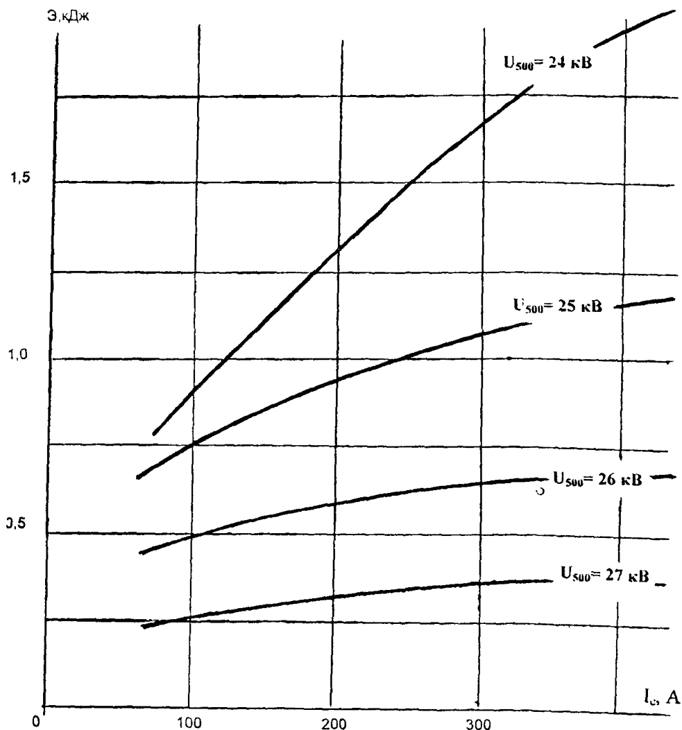
Рис.2 Обобщенные расчетные зависимости рассеиваемой ограничителем энергии за один цикл гашение-зажигание ( \mathcal{E}_1 ) в кабельной сети 10 кВ от емкостного тока однофазного замыкания на землю ( I_c ) и параметра ограничителя U_{500} .
