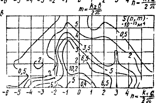
Рис. 5. Сечение двумерных спектральных плотностей полей прогибов оболочки: а - начальных; б, в - полных ( q = 0,42 q_{кр} , q = 0,8 q_{кр} )
