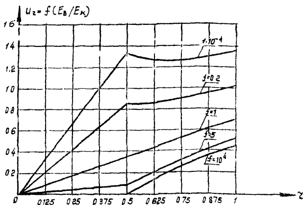
Рис. 4.5. Графики радиальных перемещений в составной круговой пластине при F_k = 1 кПа, \nu_k = \nu_g = 0,3 , F_g = 10000., 5., 1., 0.2, 0.0001 кПа
