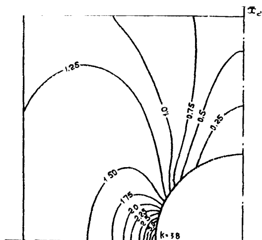
Рис. 5.25. Изолинии \sigma_{zz} при \rho = 0.125(R_H + 7R_{BH})
