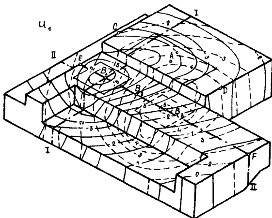
Рис. 5.31. Изолинии перемещений
