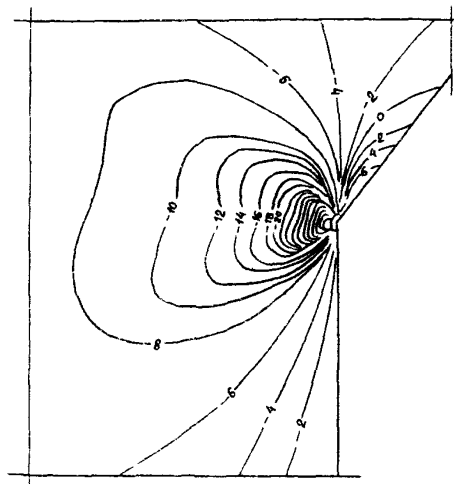
Рис. 5.14. Изолинии напряжений \sigma_{22} у опорной пяты свода
