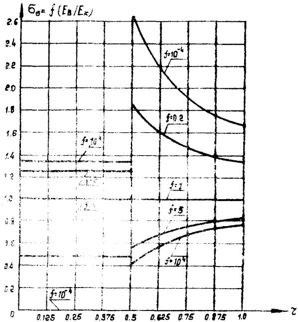
Рис. 4.7. Графики кольцевых напряжений в составной круговой пластине при E_K = 1 кПа, \nu_K = \nu_\theta = 0.3 , E_\theta = 0.0001, 0.2, 1, 5, 10000 кПа
