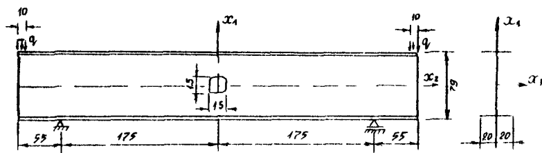
Рис. 5.6. Двутавровая балка, ослабленная отверстием
