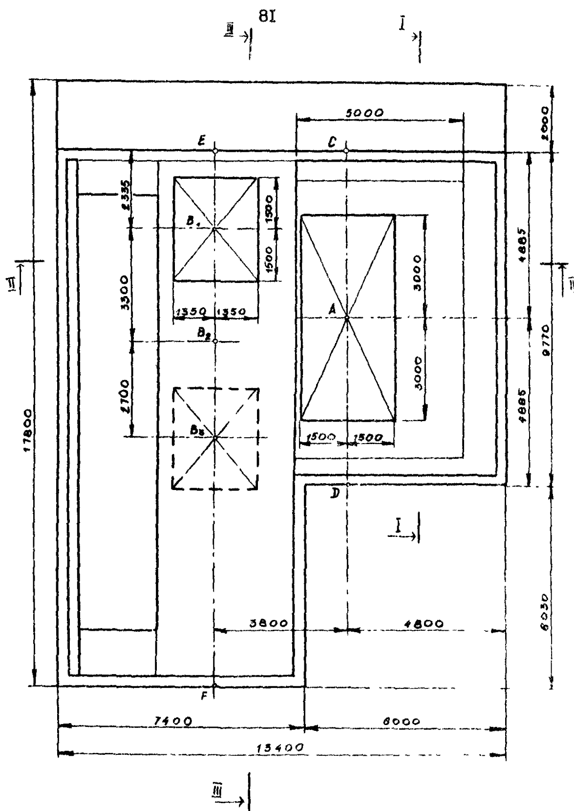
Рис. 5.28. План фундамента
