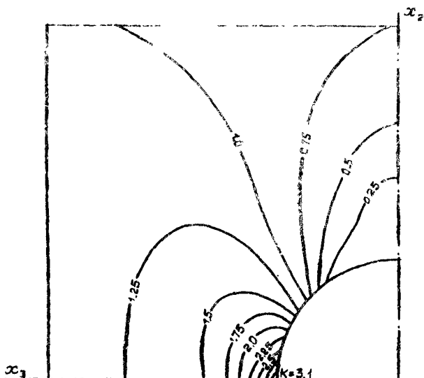
Рис. 5.17. Изолинии напряжений \sigma_{22} у отверстия в задаче Лява
