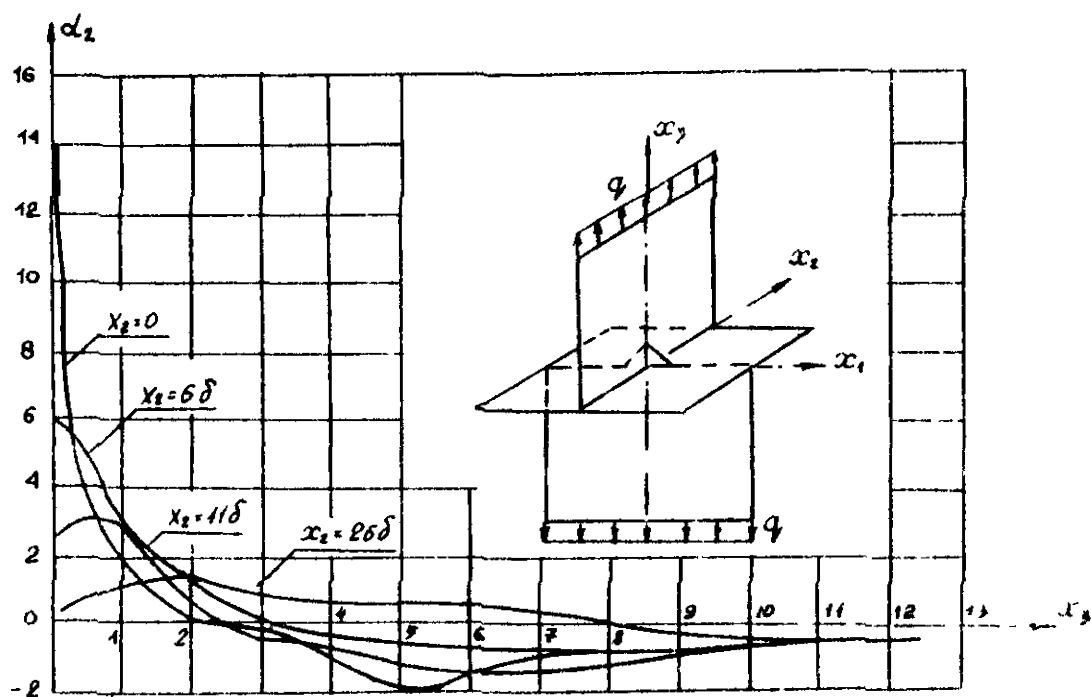
Рис. 5.10. Эпюры \alpha_2 = \sigma_{22}/q вдоль оси X_3 , при наличии трещины
