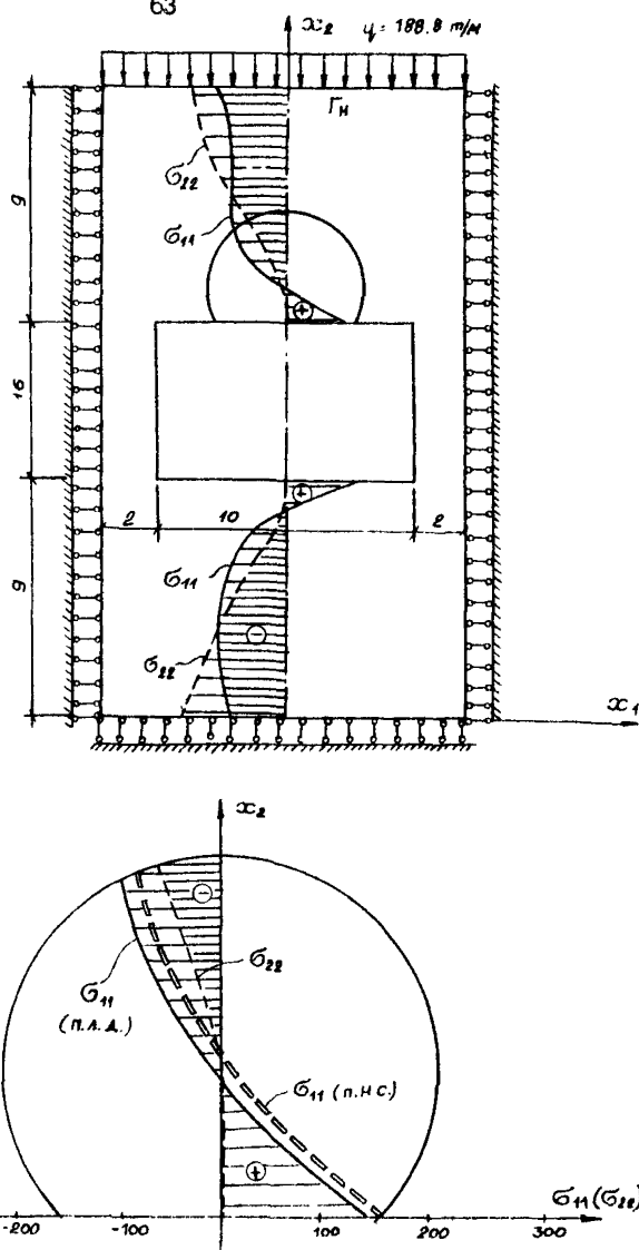
Рис. 5.12. Эпюры нормальных напряжений \sigma_{11} и \sigma_{22} в массиве горных пород, ослабленном выработкой
