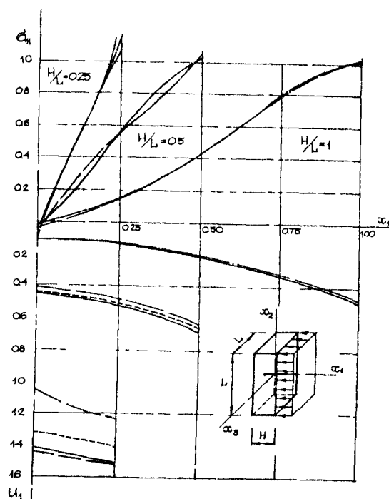
Рис. 4.3. Напряжение \sigma_{II} и перемещение u_1 в толстой пластине при x_L - x_s = 0
