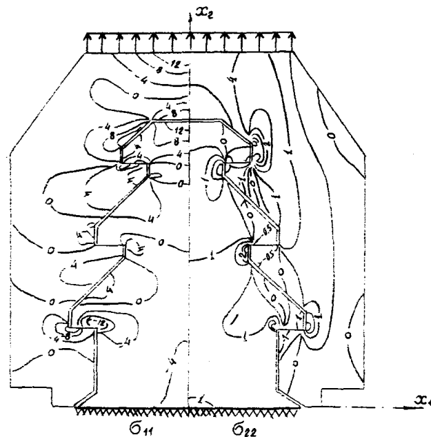
Рис. 5.3. Изолинии нормальных напряжений в хвостовом соединении
