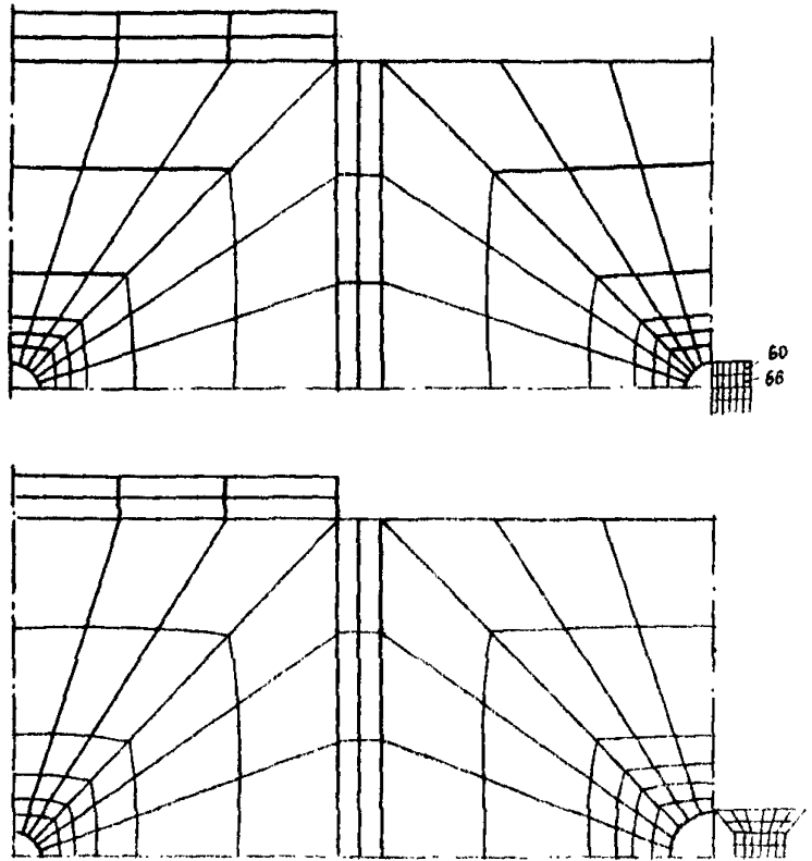
Рис. 5.16 Фрагментация граничной поверхности
