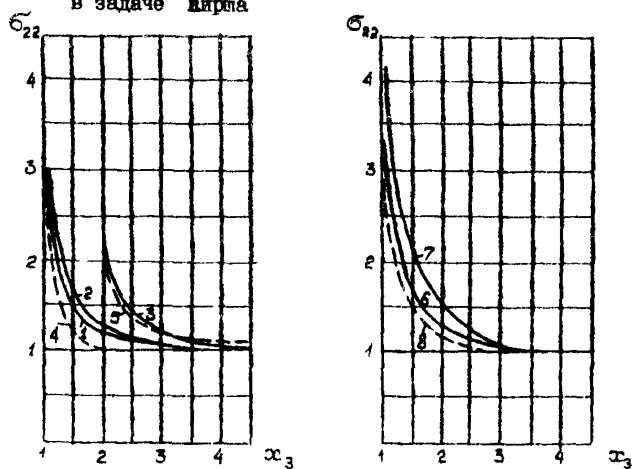
Рис. 5.18. Изменение напряжений \sigma_{22} у отверстия в плоскости x_1 - O
