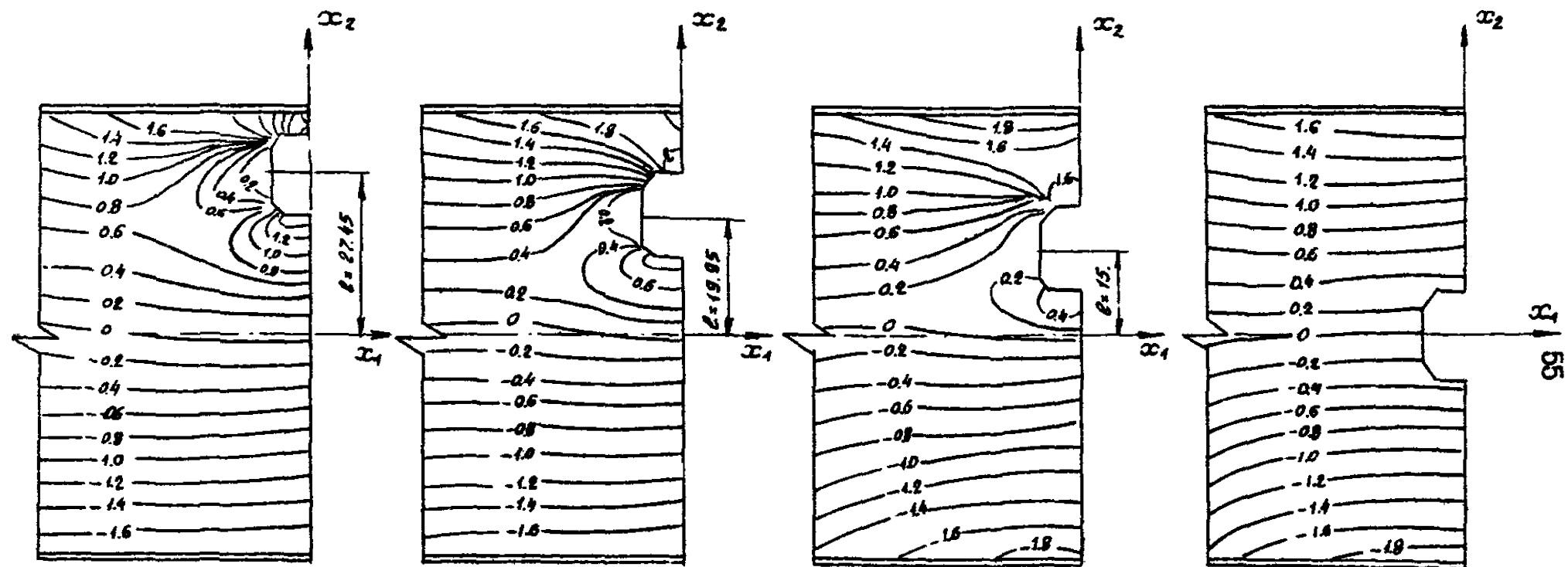
Рис. 5.8. Изолинии напряжений \sigma_{11}
