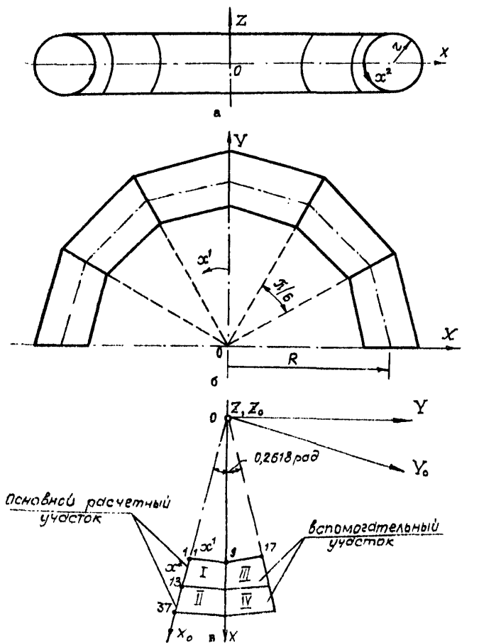
а, б – общий вид оболочки; в – расчетный фрагмент оболочки Рис. 4.9
