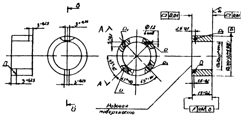
Черт. 4. Неполаякий образец машины УМТ-1
