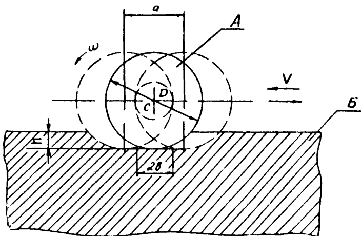
черт. 3. Схема взаимодействия образцов на машине трения А-2
