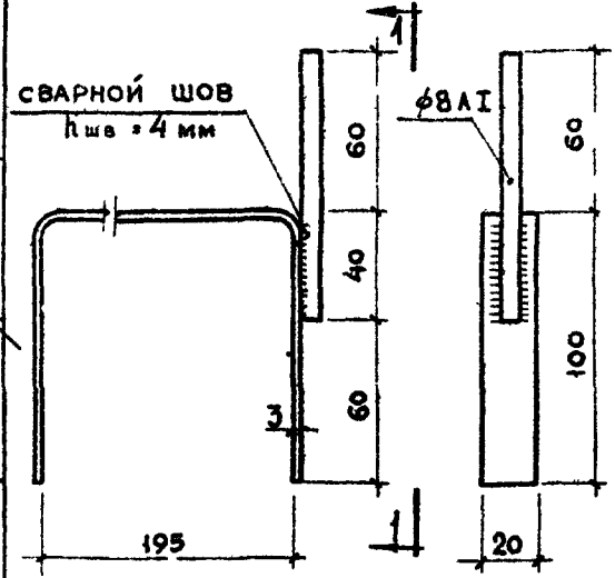
СКОБА С АНКЕРОМ
