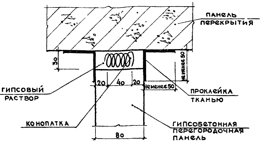
МЕЖДУКОМНАТНАЯ ПЕРЕГОРОДКА
