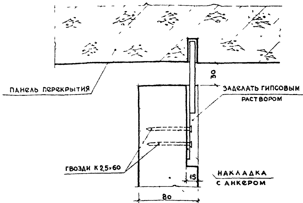
ГИПСОБЕТОННАЯ ПЕРЕГОРОДОЧНАЯ ПАНЕЛЬ
