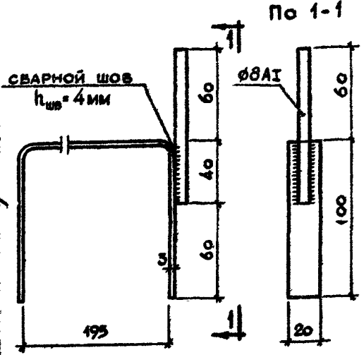
СКОБА С АНКЕРОМ
