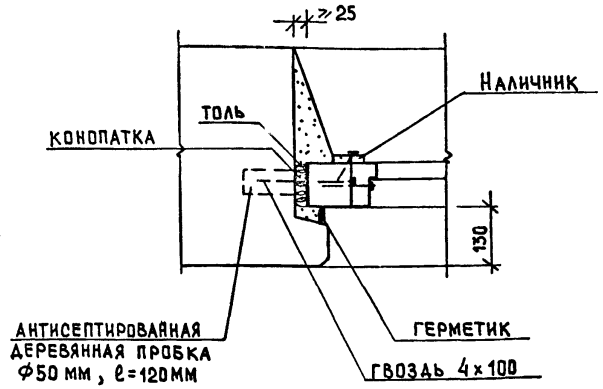
Боковое сечение
