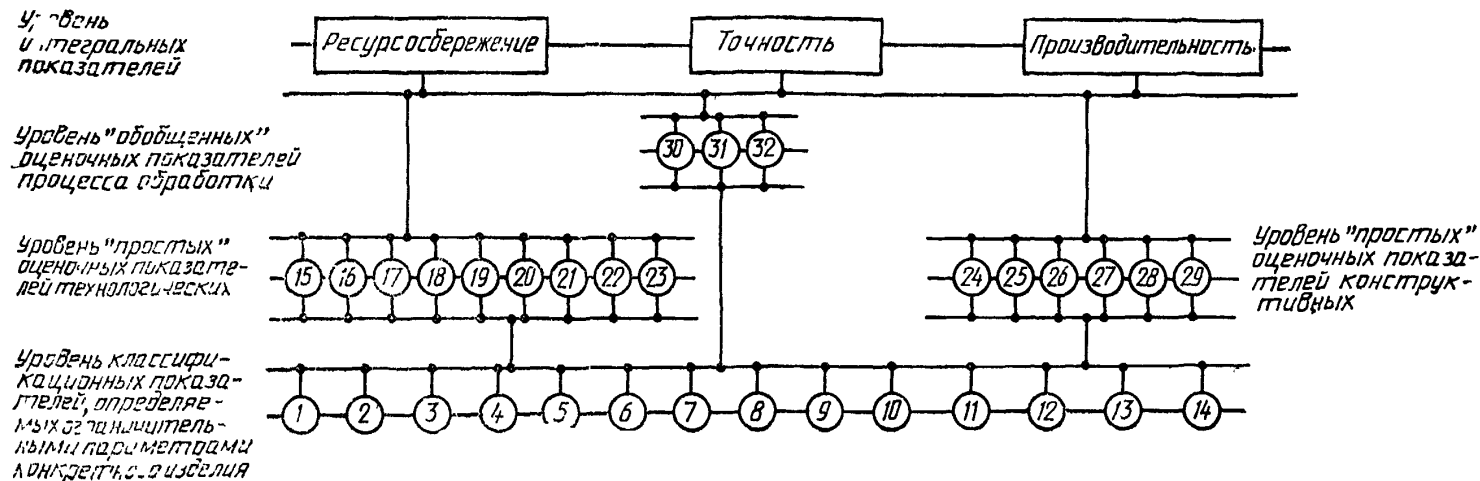
Рис. 3.6. Информационная модель для сравнительного анализа технологических наладок круглошлифовальных станков:
