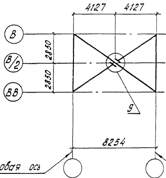
Фрагмент 1 М 1:200
