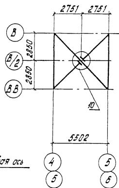
Фрагмент 2 М 1:200
