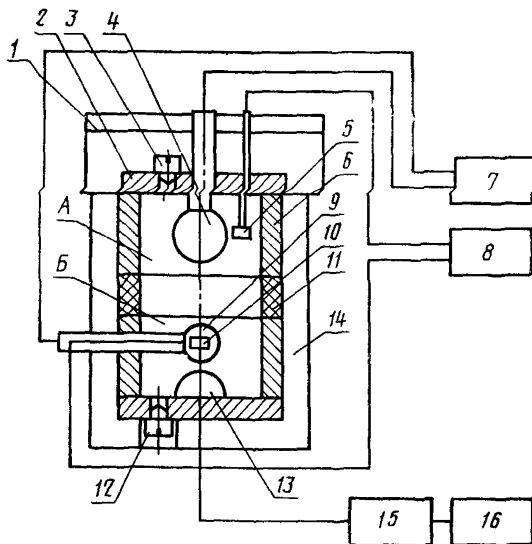
Установка для измерения чувствительности гидрофона:
