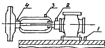
Горизонтальное положение оси клапана по отношению к платформе и параллельное по отношению к магистральным фланцам корпуса
