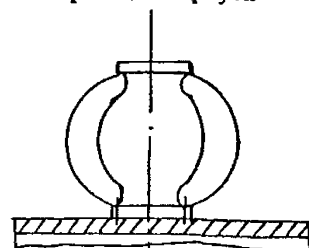
Горизонтальное положение оси клапана по отношению к платформе и параллельное по отношению к магистральным фланцам корпуса
