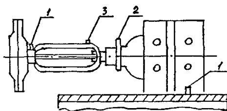
Горизонтальное положение оси клапана по отношению к платформе и перпендикулярное по отношению к магистральным фланцам корпуса
