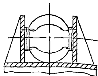
Горизонтальное положение оси клапана по отношению к платформе и перпендикулярное по отношению к магистральным фланцам корпуса
