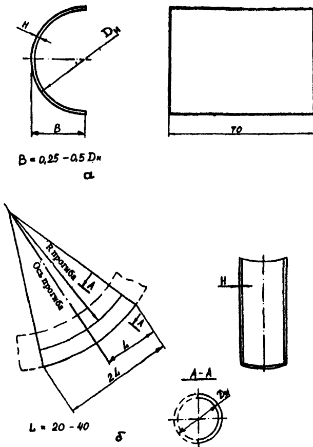
Рис. ПА.2- СОП в виде фрагментов изделий: а - отрезок трубы; б - участкагиба трубы; D_{\text{н}} - номинальный диаметр; H - толщина стенки
