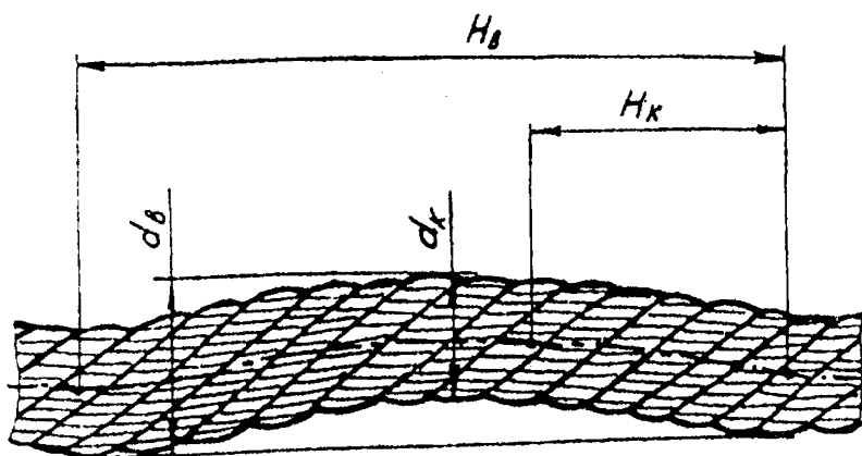
Рис. 12. Волнистость каната
