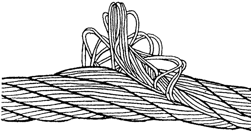
Рис. 10. Выдавливание сердечника
