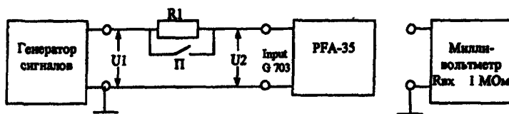
Рисунок 5. Измерение входного сопротивления прибора.
