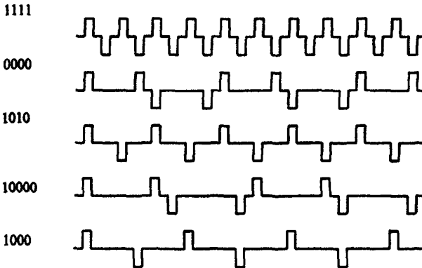
Рисунок 3. Формирование кода сигнала HDB-3.
