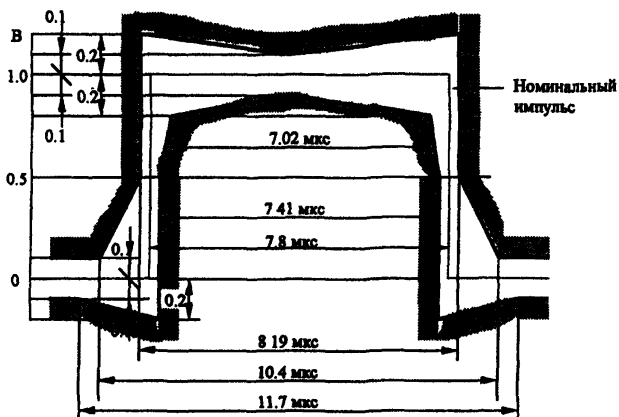
Рисунок 2а. Шаблоны импульсов для сонаправленного стыка (64 кбит/с).
