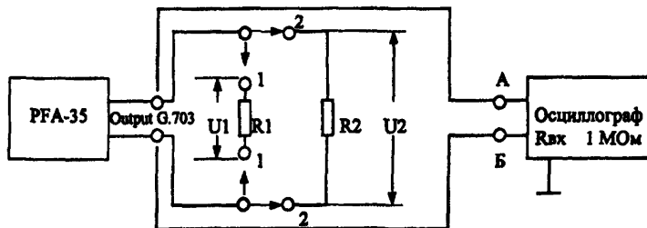
Рисунок 4 Схема измерения выходного сопротивления прибора
