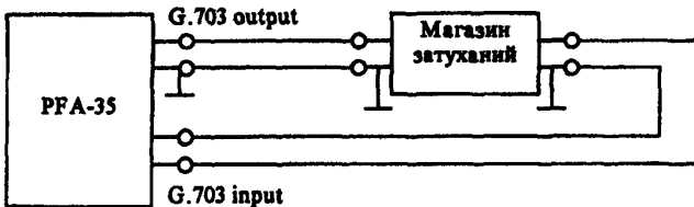
Рисунок 8. Измерение чувствительности приемника на входе G.703
