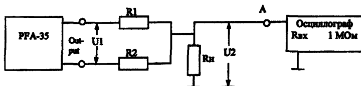
Рисунок 6 Измерение затухания асимметрии выхода прибора
