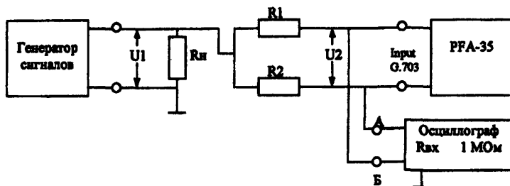
Рисунок 6 Измерение затухания асимметрии выхода прибора
