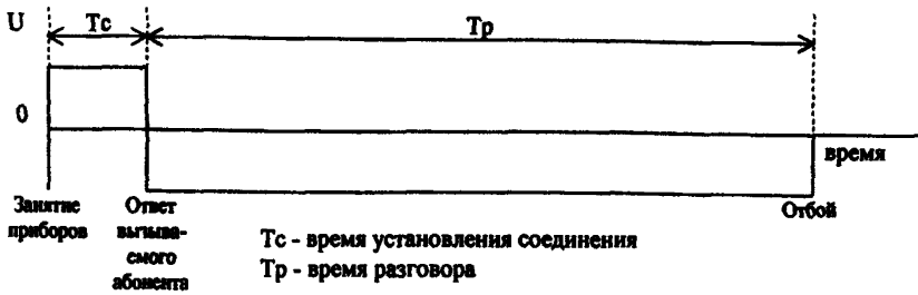
Рисунок 4 - Однократная переполусовка напряжения станционной батареи при ответе вызываемого абонента
