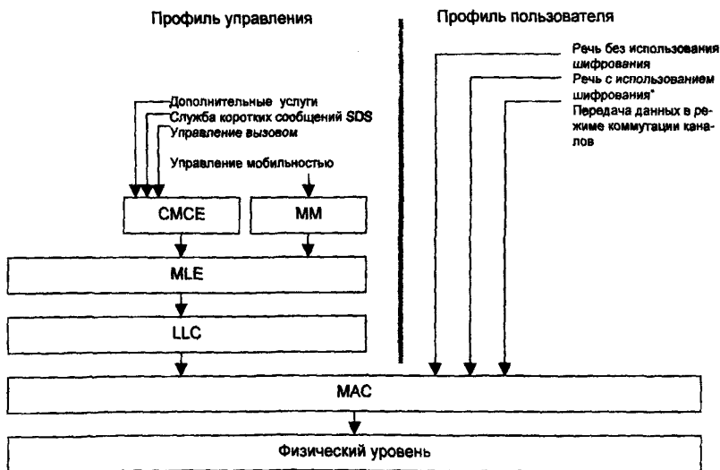
Рисунок 2 - Архитектура радиоинтерфейса TETRA V+D
