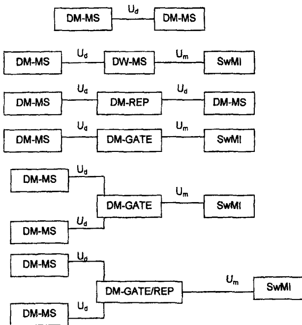
Рисунок 1б - Варианты организации связи в сети TETRA с использованием DMO
