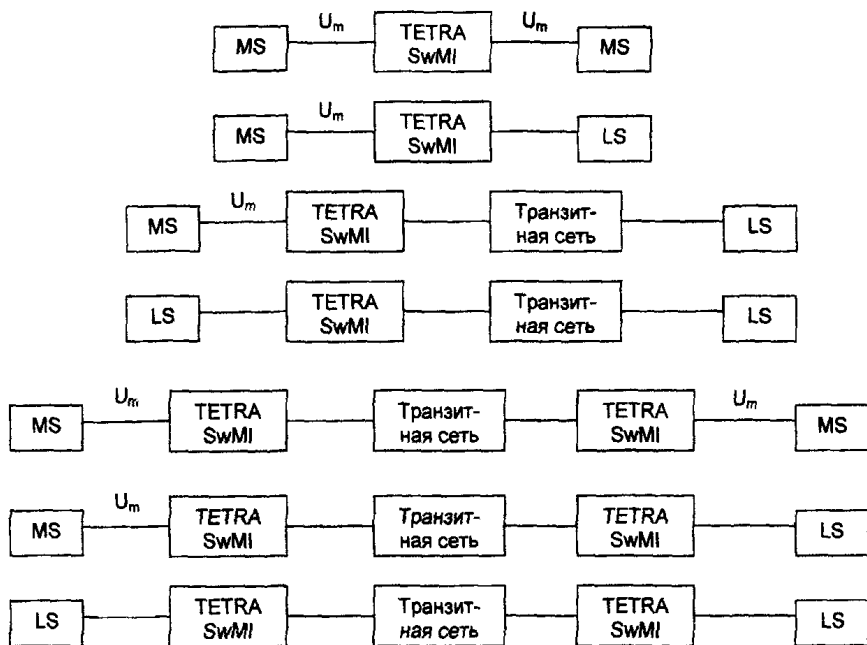
Рисунок 1а - Варианты организации связи в сети TETRA (V+D).
