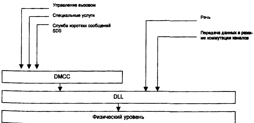
Рисунок 3 - Архитектура радиоинтерфейса TETRA DMO
