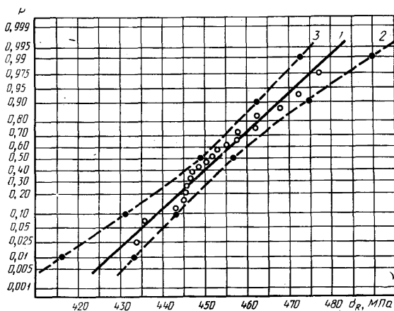
90 %-ная доверительная область распределения предела прочности образцов из дюралюминиевого профиля на нормальной вероятностной сетке
