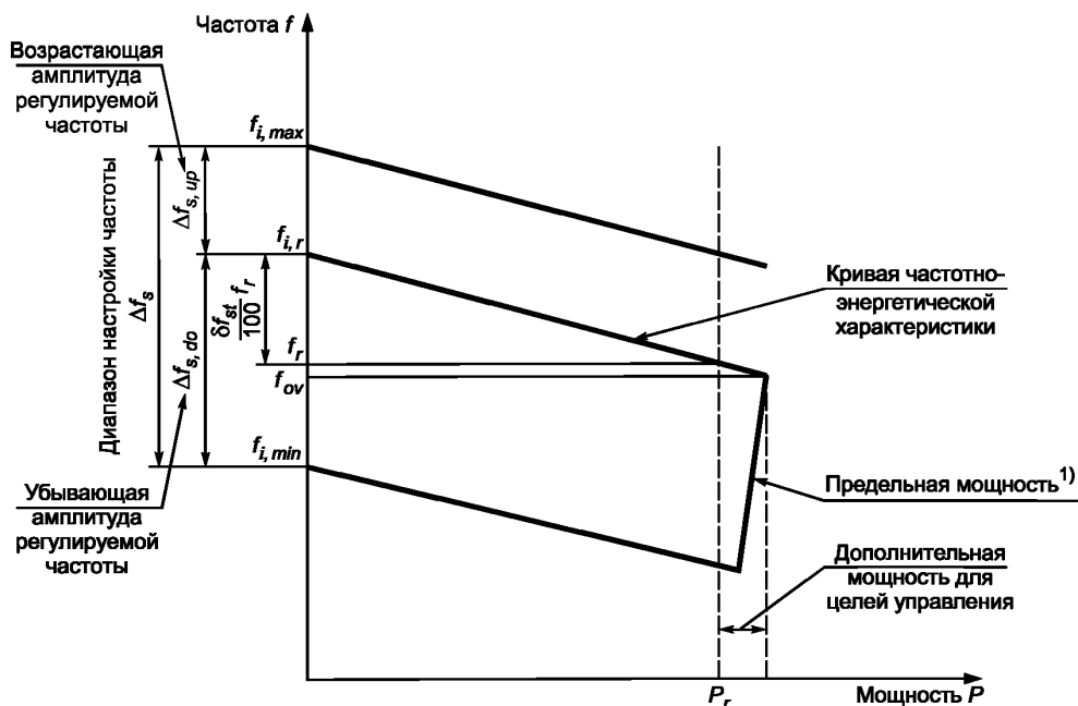
Рисунок 1 — Частотно-энергетическая характеристика диапазона регулируемой частоты
