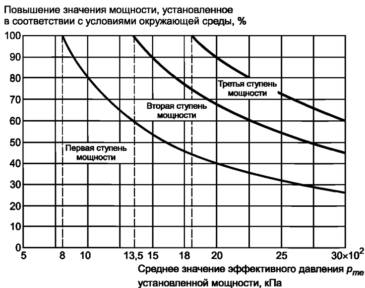
Рисунок 8 — Ориентировочные значения внезапного максимального повышения мощности как функции тормозного эффективного среднего значения давления p_{me} при объявленной мощности (четырёхтактные двигатели)
