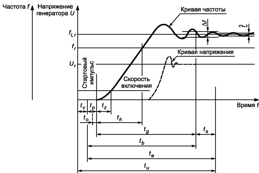
Рисунок 10 — Пусковые характеристики
