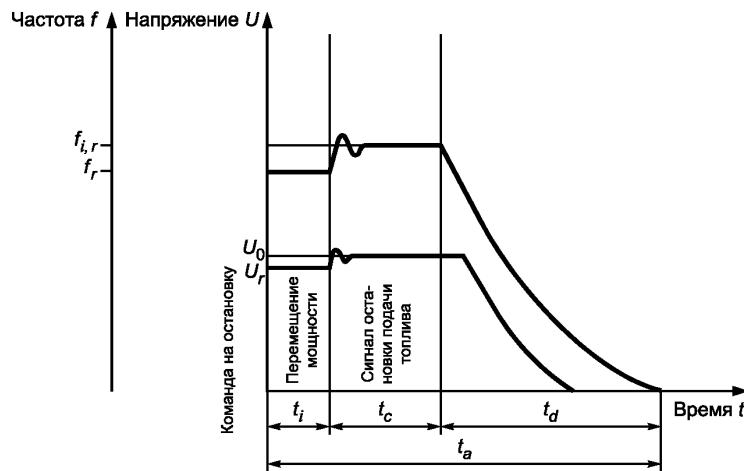
Рисунок 11 — Характеристики остановки
