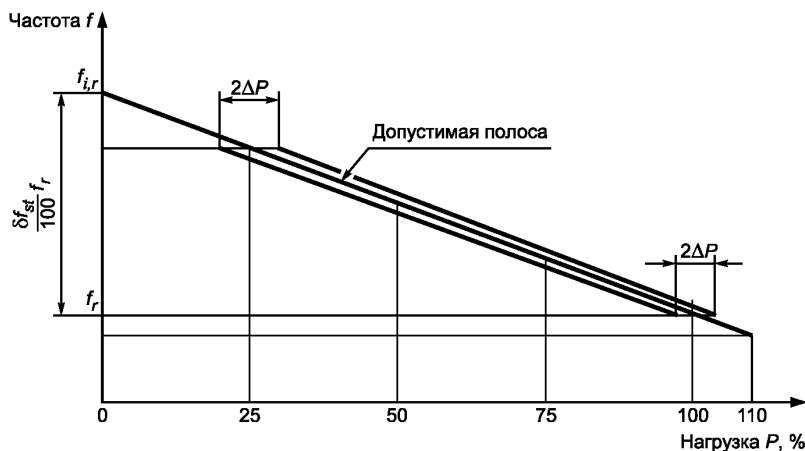
Рисунок 12 — Распределение мощности при параллельной нагрузке
