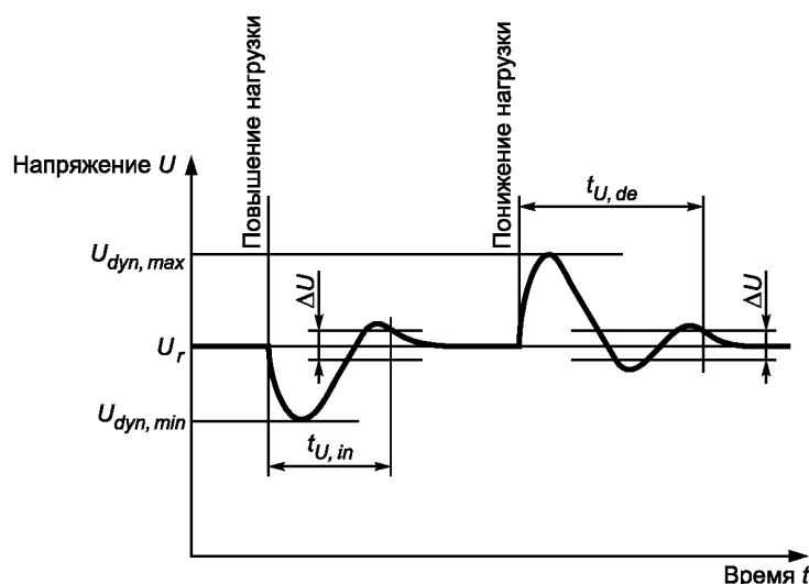
Рисунок 5 — Характеристики кратковременного напряжения без квадратурнотекущего статического отклонения напряжения компенсации
