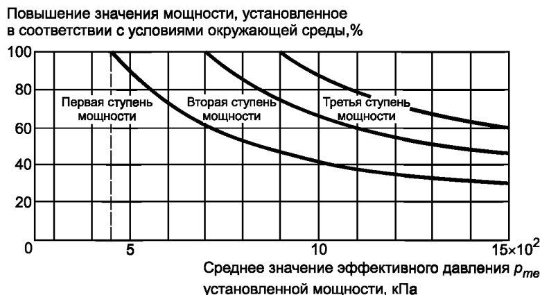
Рисунок 9 — Ориентировочные значения внезапных максимальных повышений мощности как функции тормозного эффективного среднего значения давления p_{me} при объявленной мощности (двухтактные высокоскоростные двигатели)
