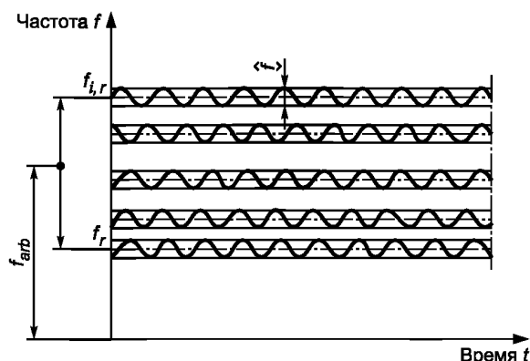
Рисунок 3 — Стабилизированная полоса частот
