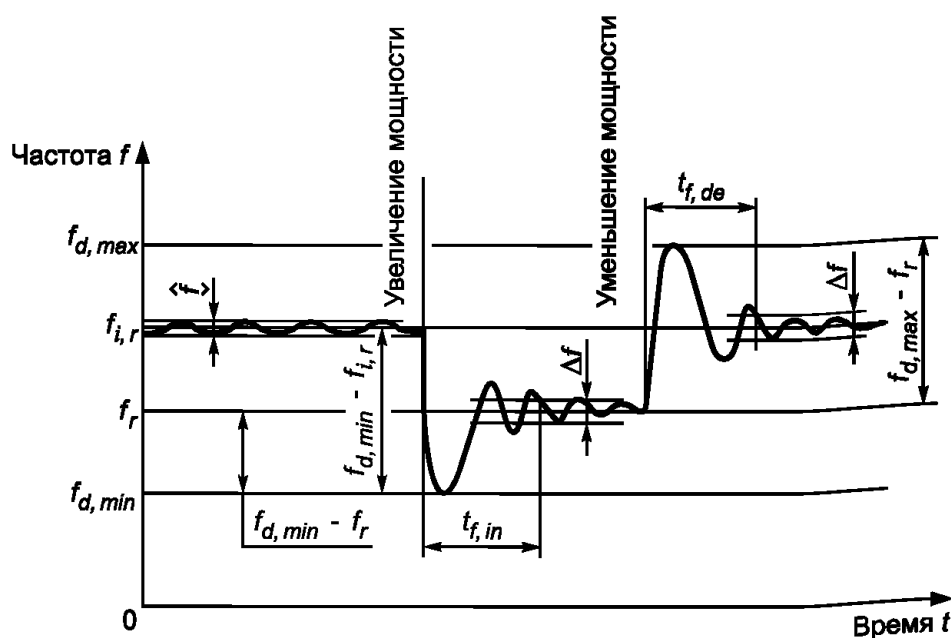
Рисунок 4 — Динамический режим частоты
