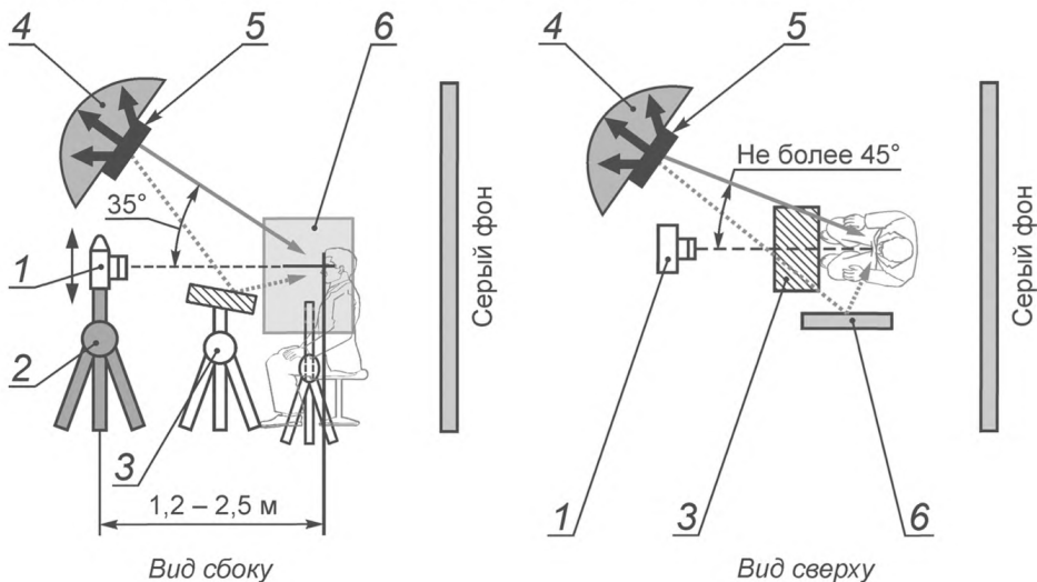
Рисунок Б.4 — Организация освещения фотолаборатории с использованием одного источника освещения
