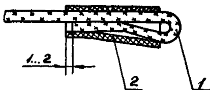
1 - провод запаса; 2 - электроизоляционная трубка
