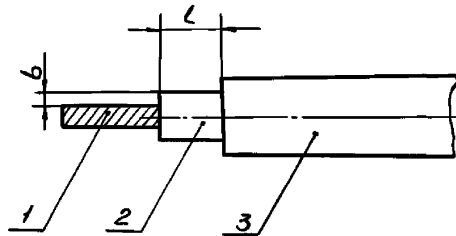
1 - жила; 2 - изоляция; 3 - защитный покров
