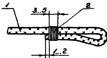
1 - провод запаса; 2 - бандаж из ниток
