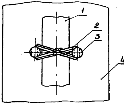
1 - жгут; 2 -шнур; 3 - стойка (винт); 4-панель
