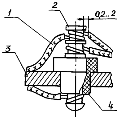
1 - провод; 2 - цилиндрический контакт; 3 - плата; 4 - втулка
