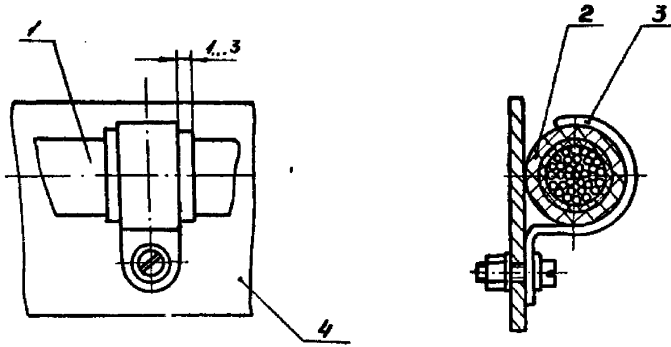
1 - жгут; 2 - электроизоляционная прокладка; 3 - скоба; 4 - панель
