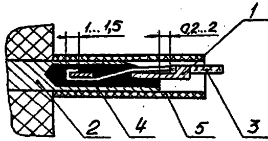
1-наконечник; 2-контакт соединителя; 3-провод; 4 - припой; 5- электроизоляционная трубка.
