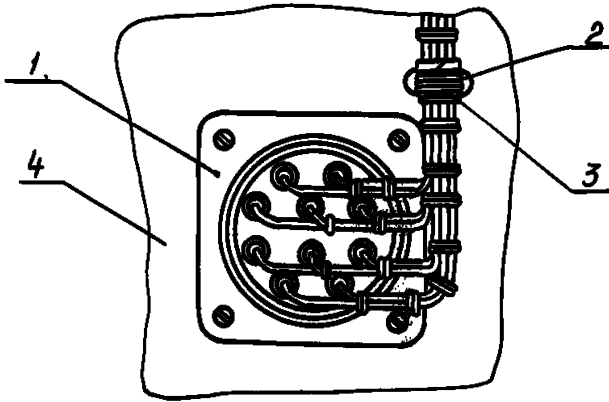
1-соединитель; 2-отверстие для крепления жгута; 3-нити или шнур; 4-панель.
