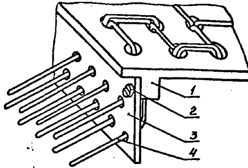
1 - матрица; 2 - винт крепления гребенки; 3 - технологическая гребенка; 4 - провод
