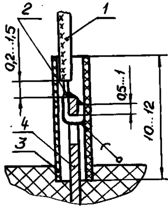
1-провод; 2- токопроводящая жила; 3- электроизоляционная трубка; 4- контакт соединителя.
