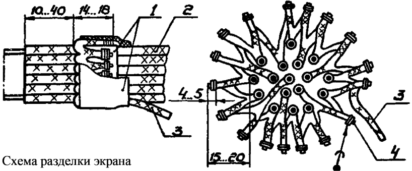
Схема соединения экранов
