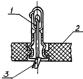
1 - плоский контакт; 2 - плата; 3 - провод
