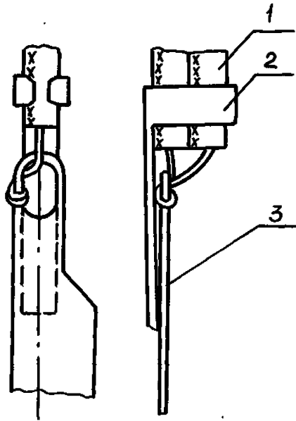
1-провод; 2-наконечник; 3-плоский контакт.
