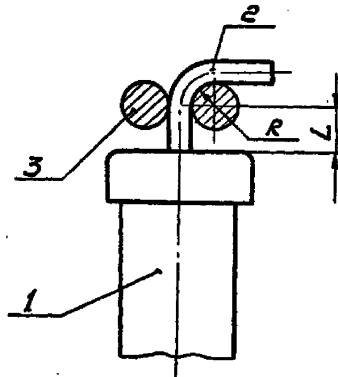
1- электрорадиоэлемент; 2- вывод; 3- приспособление для гибки; L-расстояние от корпуса элемента до центра радиуса изгиба вывода; R - радиус гибки.
