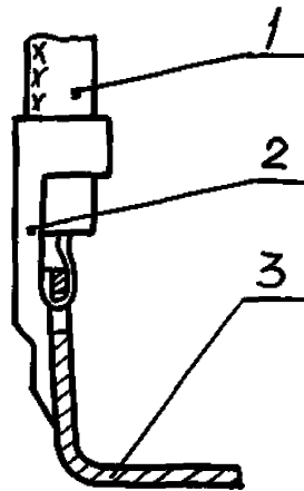
1-провод; 2-наконечник; 3-плоский контакт.
