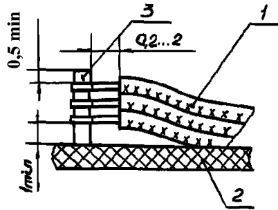
1 - провод; 2 - плата; 3 - цилиндрический контакт.
