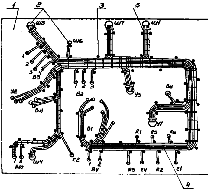
1-шаблон; 2-отверстие в шаблоне; 3-шпилька; 4-жгут; 5-шаблон-имитатор соединителя
