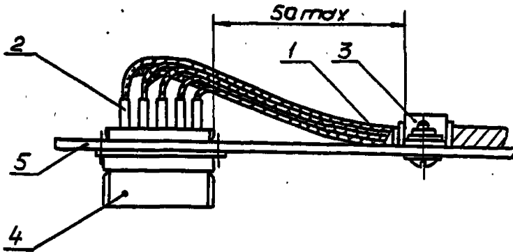
1-жгут; 2-электроизоляционная трубка; 3-скоба; 4-соединитель; 5-панель.
