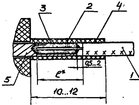
1-провод; 2-токопроводящая жила; 3-припой; 4-электроизоляционная трубка; 5-контакт соединителя типа 2PM. Величина в соответствии с 10.3.5.
