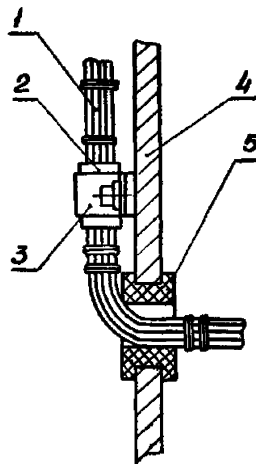
1 - жгут; 2 - электроизоляционная прокладка; 3 - скоба; 4 - панель 5-электроизоляционная втулка
