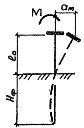
Расчетная схема
