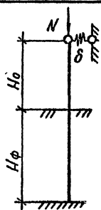
Расчетная схема для определения M
