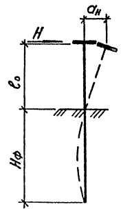
Расчётная схема
