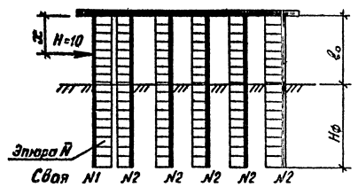
Расчетная схема
