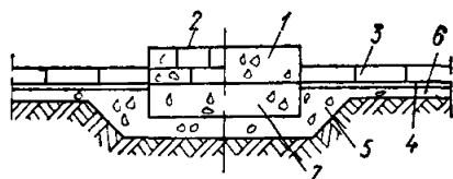
Рис. 3. Примеры фундаментов под оборудование (насосы, циркуляционные баки, опоры промывочных машин и т. д.) в отделениях электролиза водных растворов
