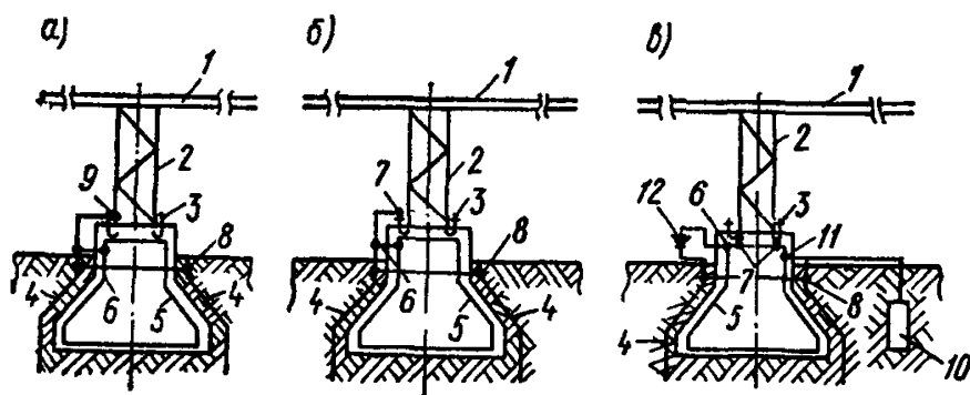
Рис. 36. Схемы экранной защиты
