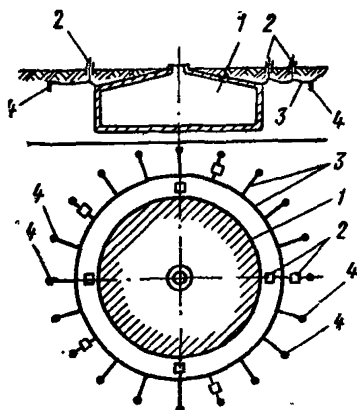
Рис. 37. Схема защиты железобетонного резервуара протекторными установками
