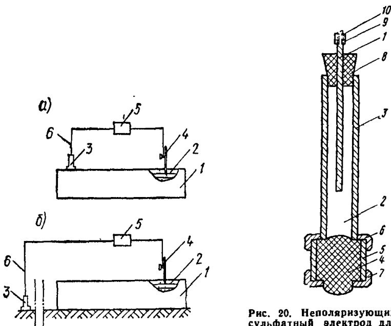
Рис. 19. Схема измерения потенциалов «арматура — бетон» (а) и «арматура — земля» (б)
