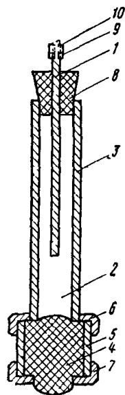
Рис. 20. Неполяризующийся медно-сульфатный электрод для контакта с бетоном
