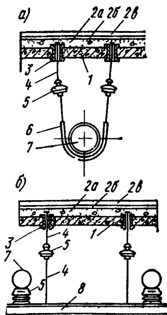
Рис. 15. Пример подвесок типа шпильки для крепления технологических трубопроводов
