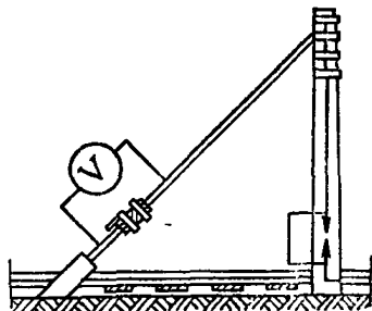
Рис. 26 Схема проверки изоляции анкеров от оттяжек опор контактной сети
