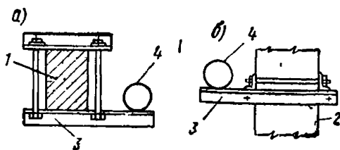
Рис. 13. Примеры выполнения держателей из электроизоляционных материалов для крепления трубопроводов
