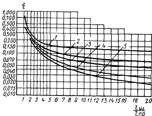
Рис 34. Номограмма для вычисления l_{ш} по \eta и \rho_{г} 1, 2, 3, 4, 5 — \rho_{г} соответственно 10, 20, 33, 100 и 200 Ом · м
