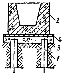
Рис. 5. Пример выполнения электроизоляционного разрыва в свайном фундаменте
