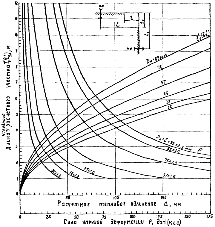
Рис. 27. Номограмма для расчета Г-образного участка трубопровода D_n = 32+89 \text{ мм}
