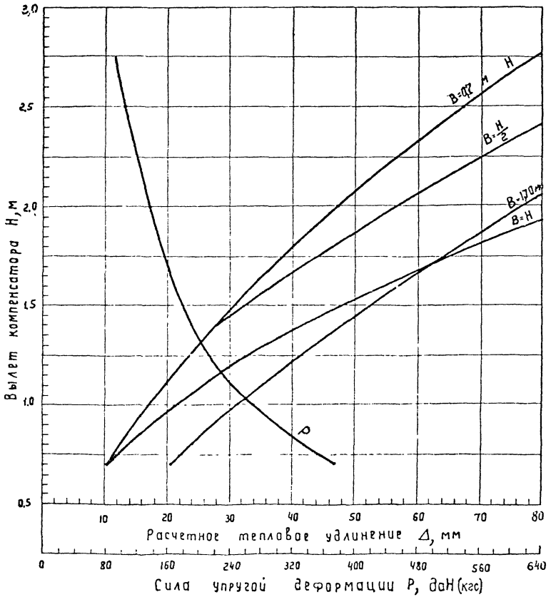
Рис.8. Номограмма для расчета П-образного компенсатора с гнутыми гладкими отводами
