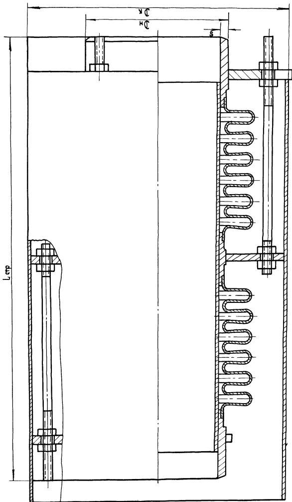
Рис. 2. Компрессор двухсекционный по ТУ 3-120-81
