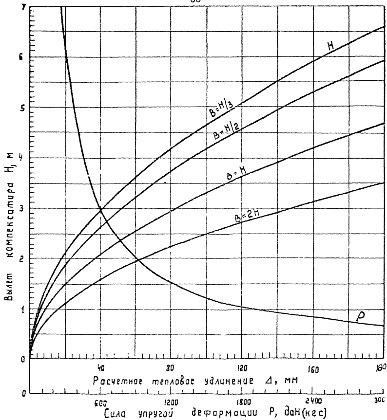
Рис.21. Номограмма для расчета П-образного компенсатора со сварными или крутоизогнутыми отводами D_H = 159 \text{ мм} , \delta = 4,5 \text{ мм}
