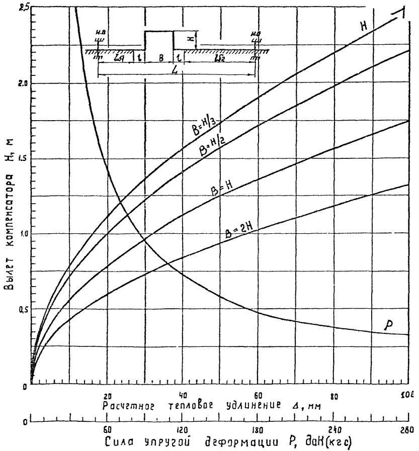
Рис.15. Номограмма для расчета П-образного компенсатора со сварными или крутоизогнутыми отводами
