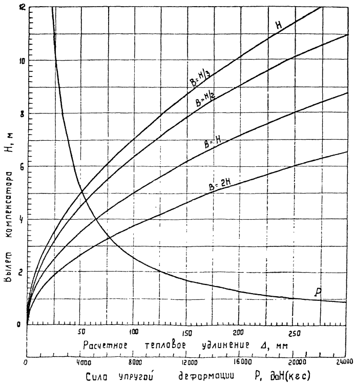
Рис.25. Номограмма для расчета П-образного компенсатора со сварными или крутоизогнутыми отводами \varnothing_n = 377 мм, \delta = 6 и 9 мм
