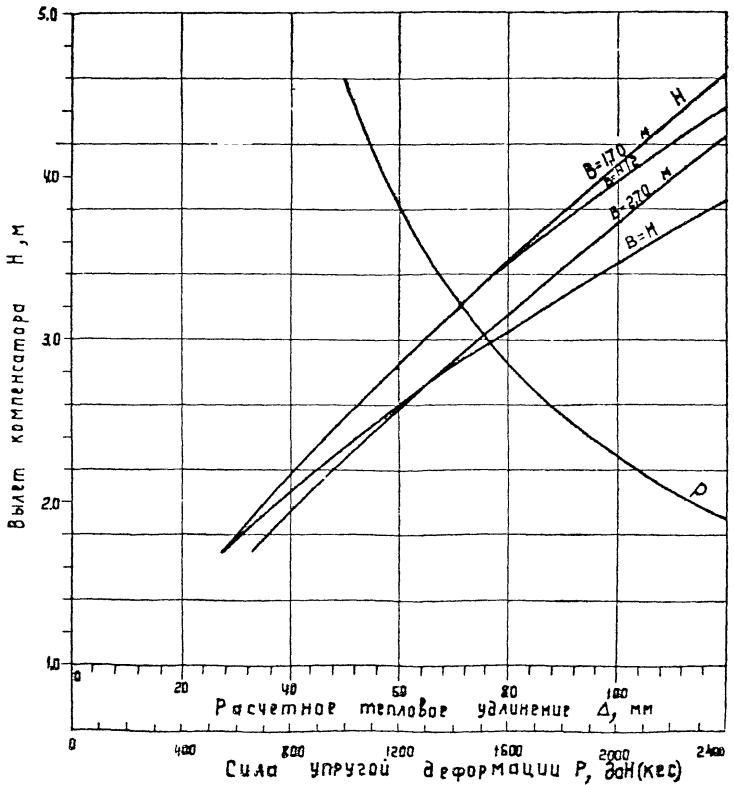
Рис.14. Номограмма для расчета П-образного компенсатора с гнутыми гладкими отводами
