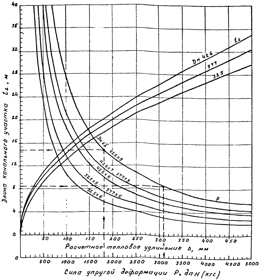
Рис.33. Номограмма для расчета Z -образного участка трубопровода Д_H = 325-426 мм
