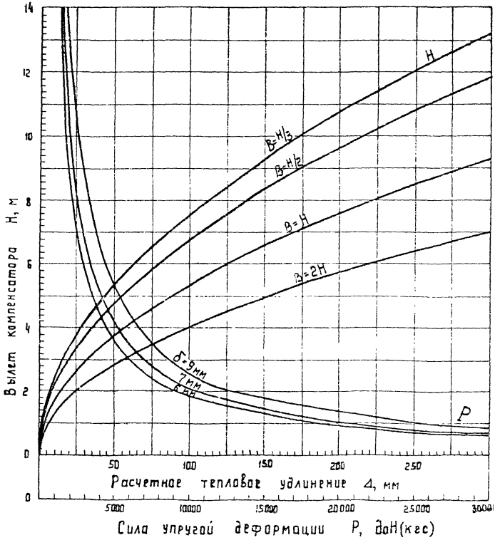
Рис.26. Номограмма для расчета U-образного компенсатора со сварными или крутоизогнутыми отводами D_H = 426 \text{ мм} , \delta = 6 \text{ и } 7 \text{ мм}
