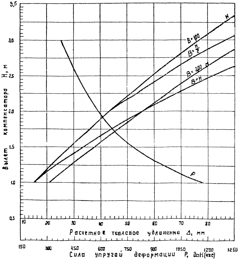
Рис.12. Номограмма для расчета П-образного компенсатора с гнутыми гладкими отводами D_H = 133 мм, \delta = 4 мм, \gamma = 0,5 м
