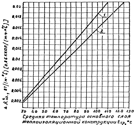
Рис. 2. График для определения величины \Delta \lambda_{из.т}^t .
