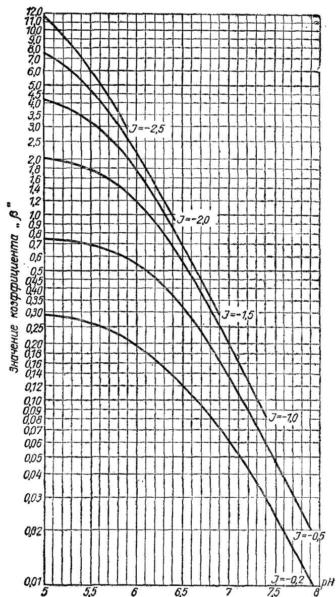
Рис. 4. График для определения дозы щелочи при pH_0 < pH_s < 8,4
