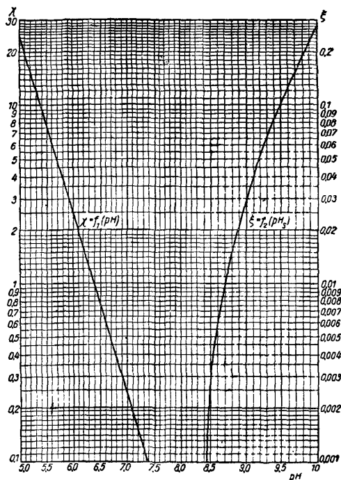
Рис. 5. График для определения дозы щелочи при \text{pH}_0 < 8,4 < \text{pH}_s
