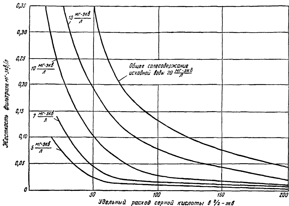
Рис. 7. График для определения жесткости воды, умягченной водород-катионированием
