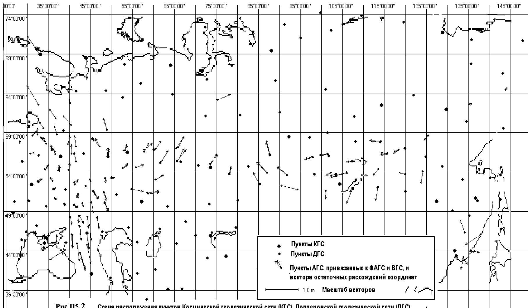
Рис.П5.2 . Схема расположения пунктов Космической геодезической сети (КГС), Доплеровской геодезической сети (ДГС) и пунктов АГС в местах расположения пунктов ФАГС и ВГС.
