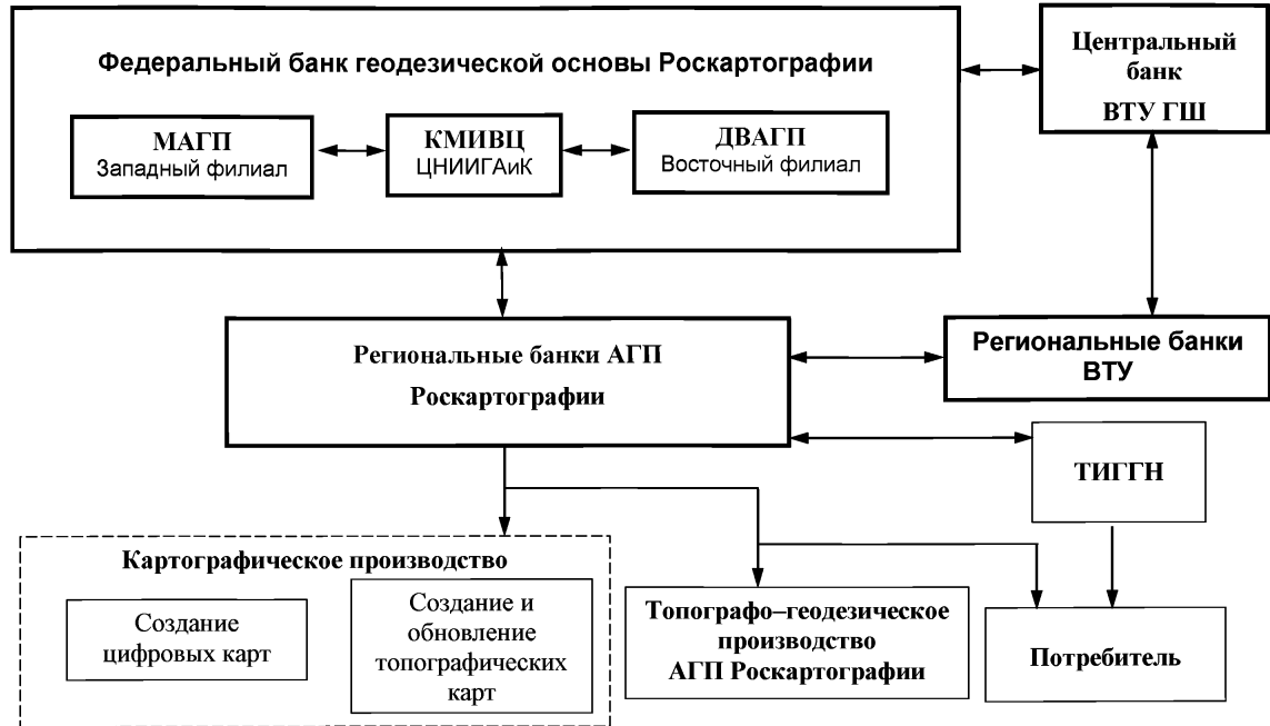
Рис. 5. Структура функционирования банков геодезической основы Роскартографии в системе топографо-геодезического и картографического производства
