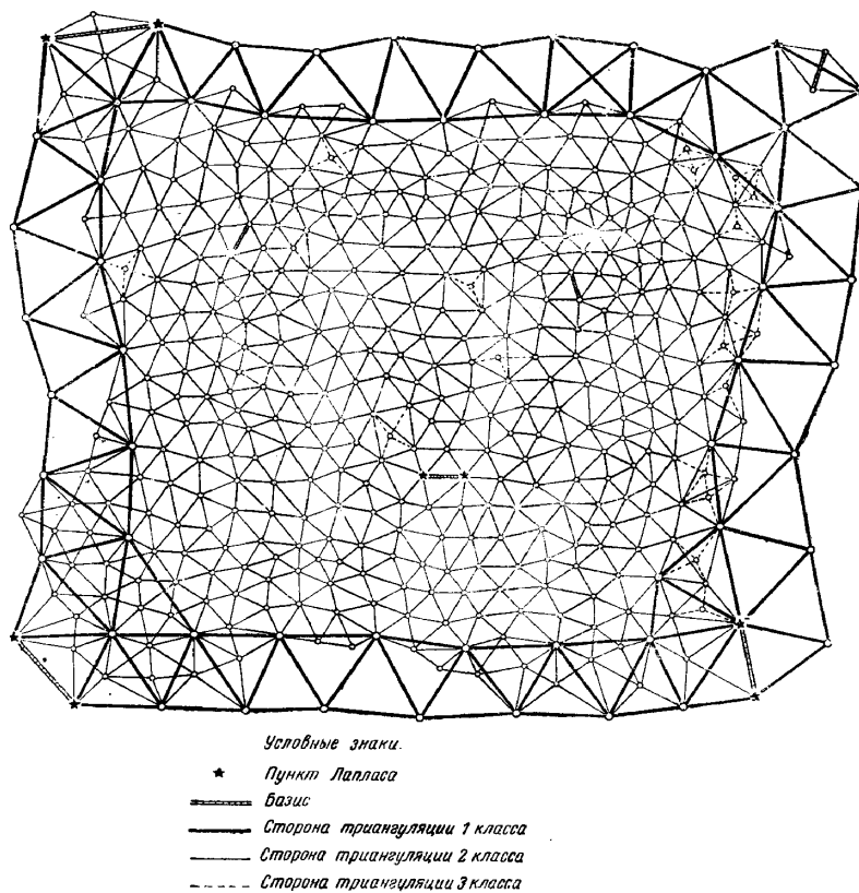
Рис.2 Схема полигона триангуляции 1 класса и заполняющей сети триангуляции 2 класса
