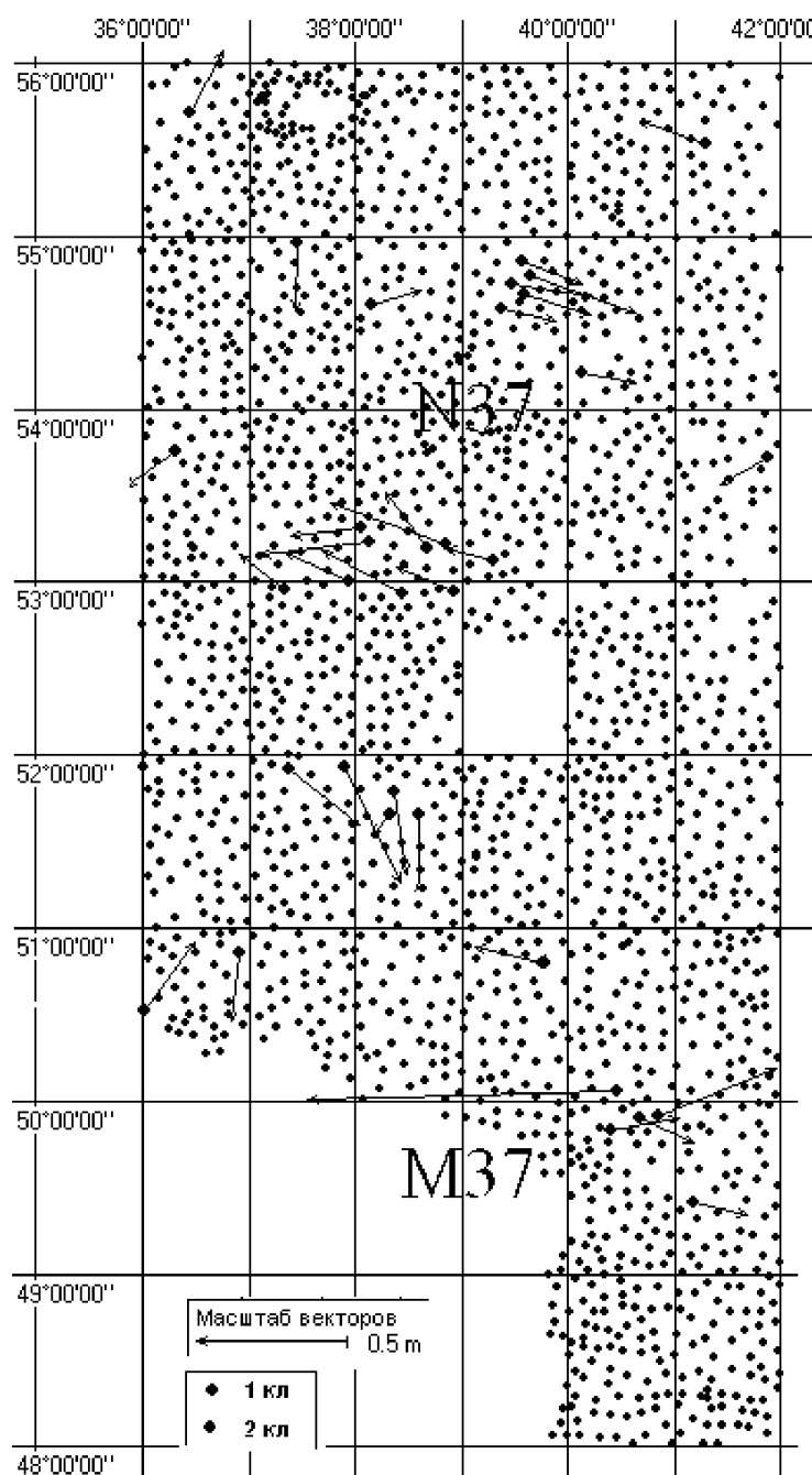
Рис П4.2 Пункты ГГС 1 и 2 классов, отображенные при построении цифровой модели преобразования координат из СК42 в СК95 на трапеции М37 и N37
