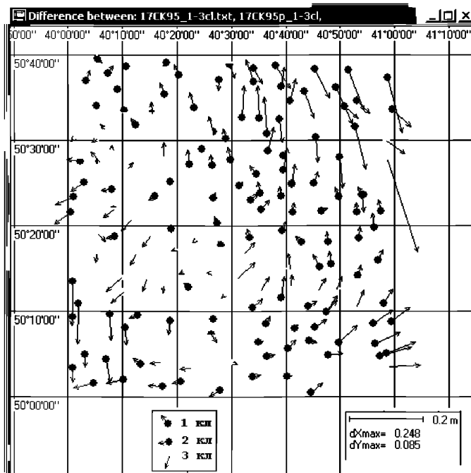
Рис. П6.6. Остаточные расхождения координат пунктов ГГС 1-3 классов при ортогональном преобразовании для трапеции М3717
