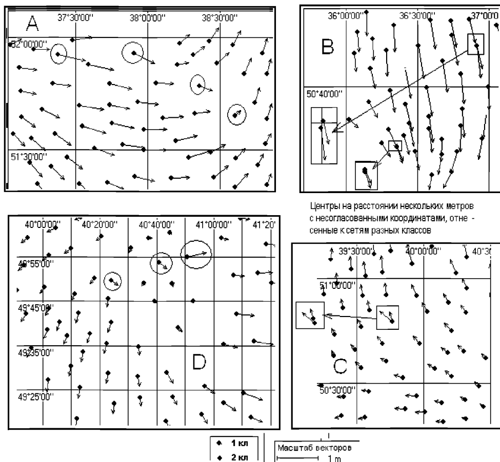
Рис. П6.2А,В,С,Д. Деформации ГГС в СК42 на отдельных участках листа М37.
