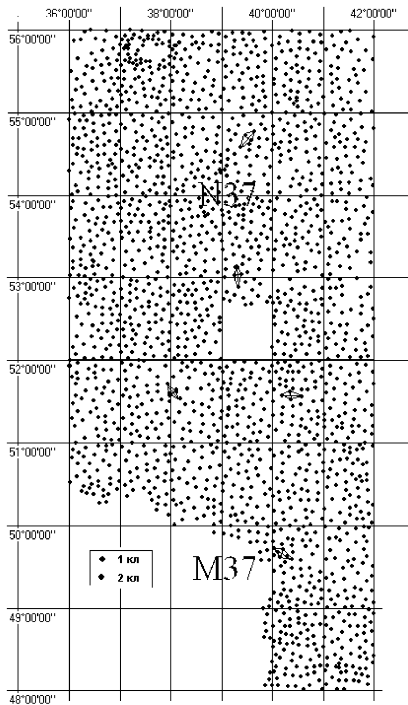
Рис. П4.1 Пункты ГГС 1 и 2 классов, использованные при построении цифровой модели преобразования координат из СК42 в СК95 на трапеции М37 и N37
