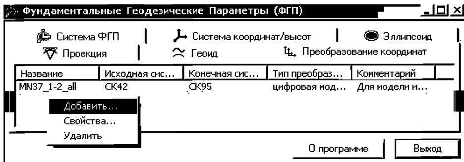
Рис. ПЗ.13 Вид окна ФГП, раздел «Преобразование координат» при внесении цифровой модели в библиотеку фундаментальных параметров
