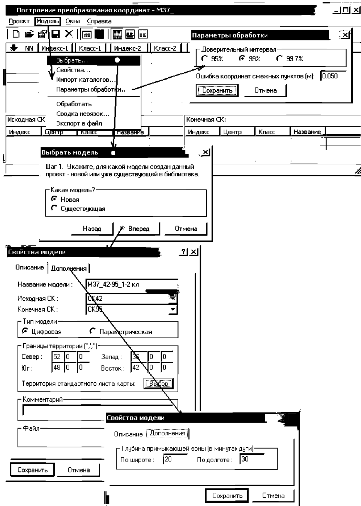
Рис. ПЗ.8 Порядок действий задания свойств модели для данной территории в двух системах координат
