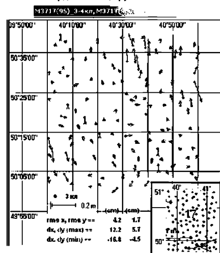
Рис. П4.66. Остаточные расхождения координат п-тов 3 класса при преобразовании координат по цифровой модели.
