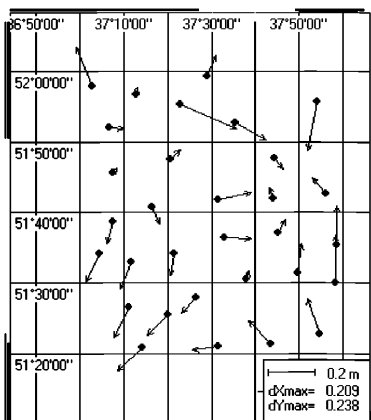
Рис. П6.4. Остаточные уклоны координат. Трапеция М3702
