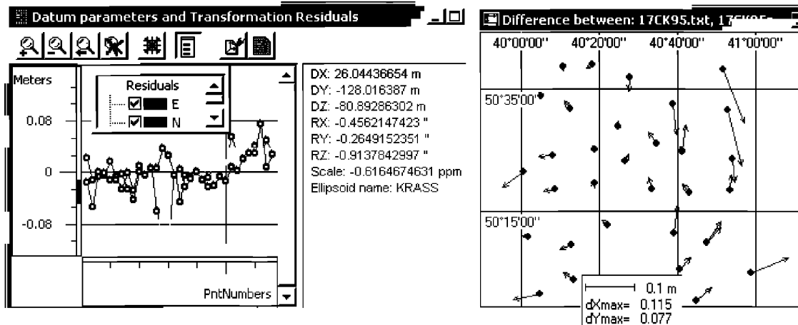
Рис. П6.5. Определение параметров преобразования для тр-ции М3717 и остаточные уклонения.
