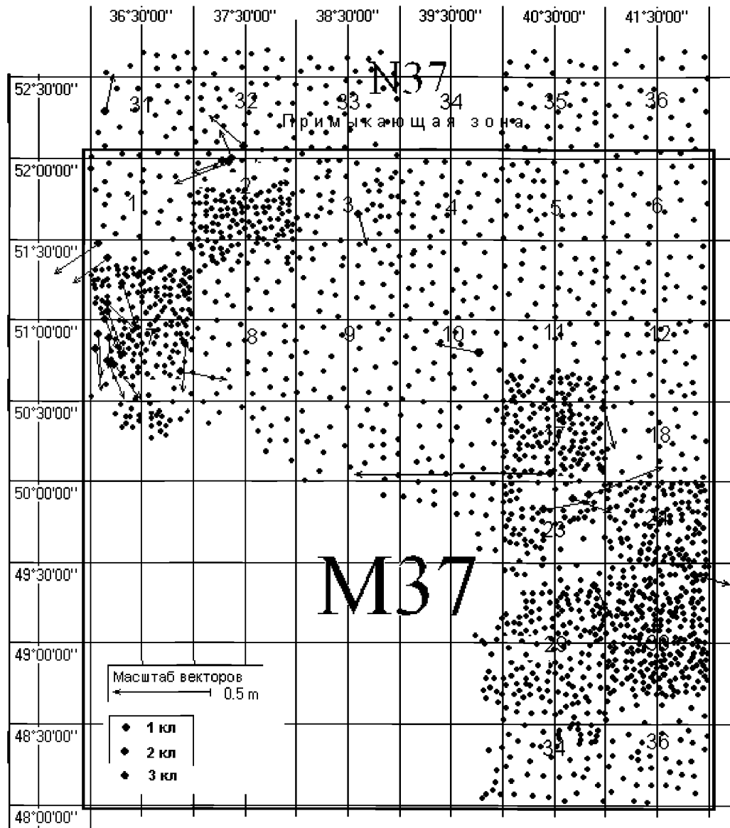
Рис. П4.3 Пункты ГГС 1, 2 и 3 классов, использованные при построении цифровой модели преобразования координат из СК42 в СК95 на трапецию М37 и вектора остаточных расхождений в положениях пунктов, данных в каталогах СК95 и полученных преобразованием по цифровой модели
