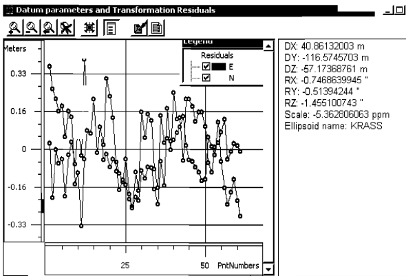
Рис. П6.3а. Определение параметров преобразования для трапеций М3702 и М3703
