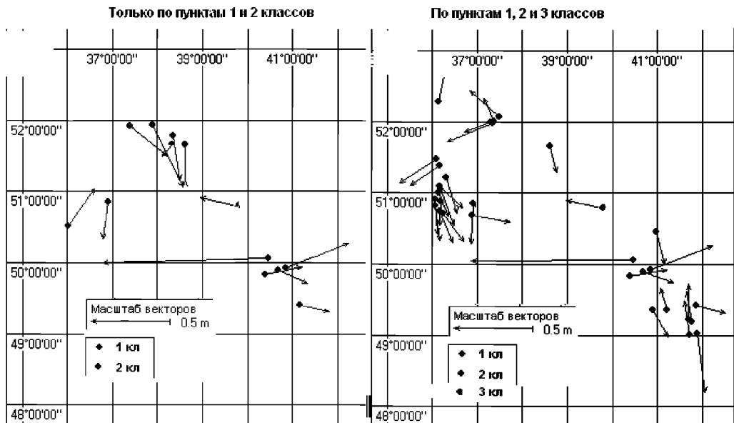
Рис. П4.4. Вектора остаточных расхождений в положениях пунктов из каталога СК-95 и полученных преобразованием из СК-42 по цифровой модели.
