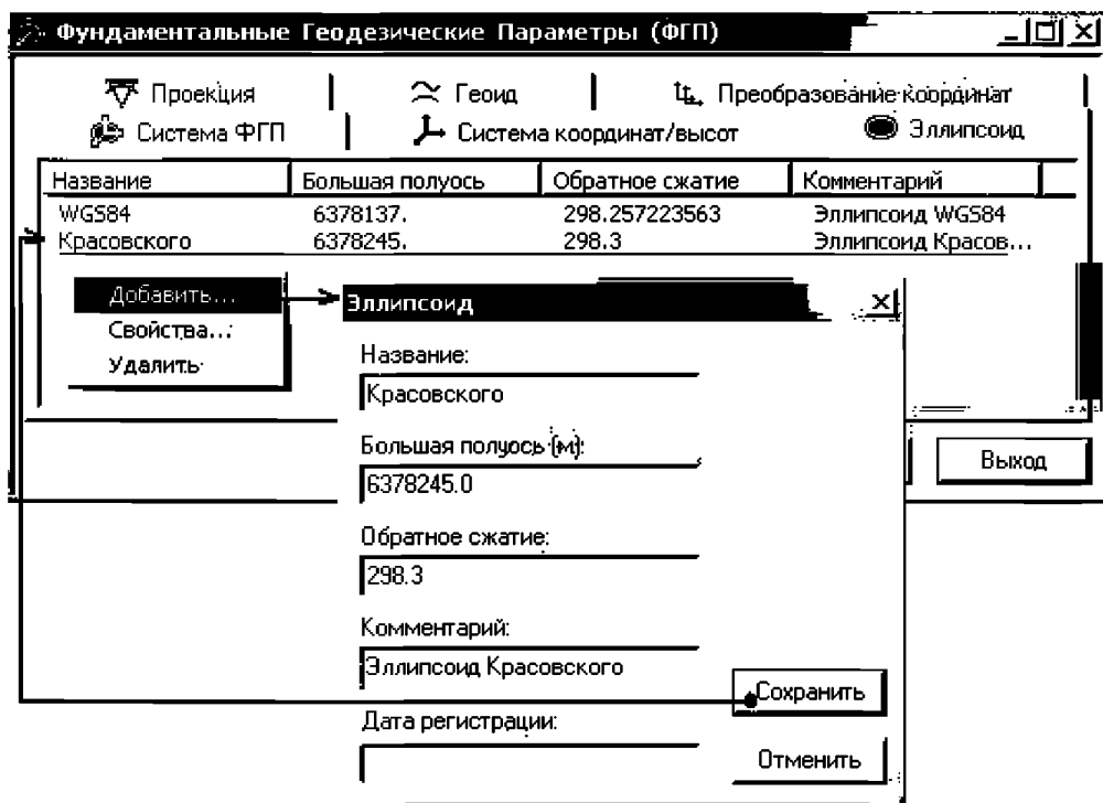
Рис. ПЗ.1 Главное окно «Фундаментальные Геодезические Параметры», закладка «Эллипсоид»
