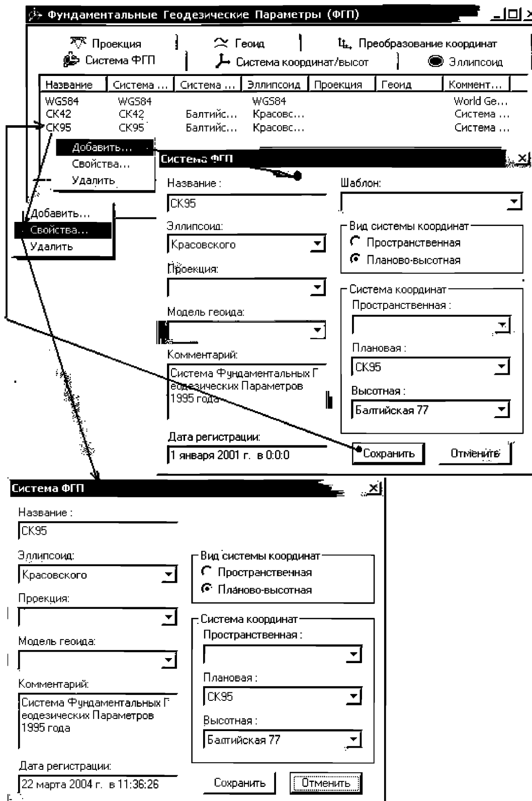
Рис. ПЗ.4 Порядок действий и содержание всех подокон при формировании ФГП для СК-95
