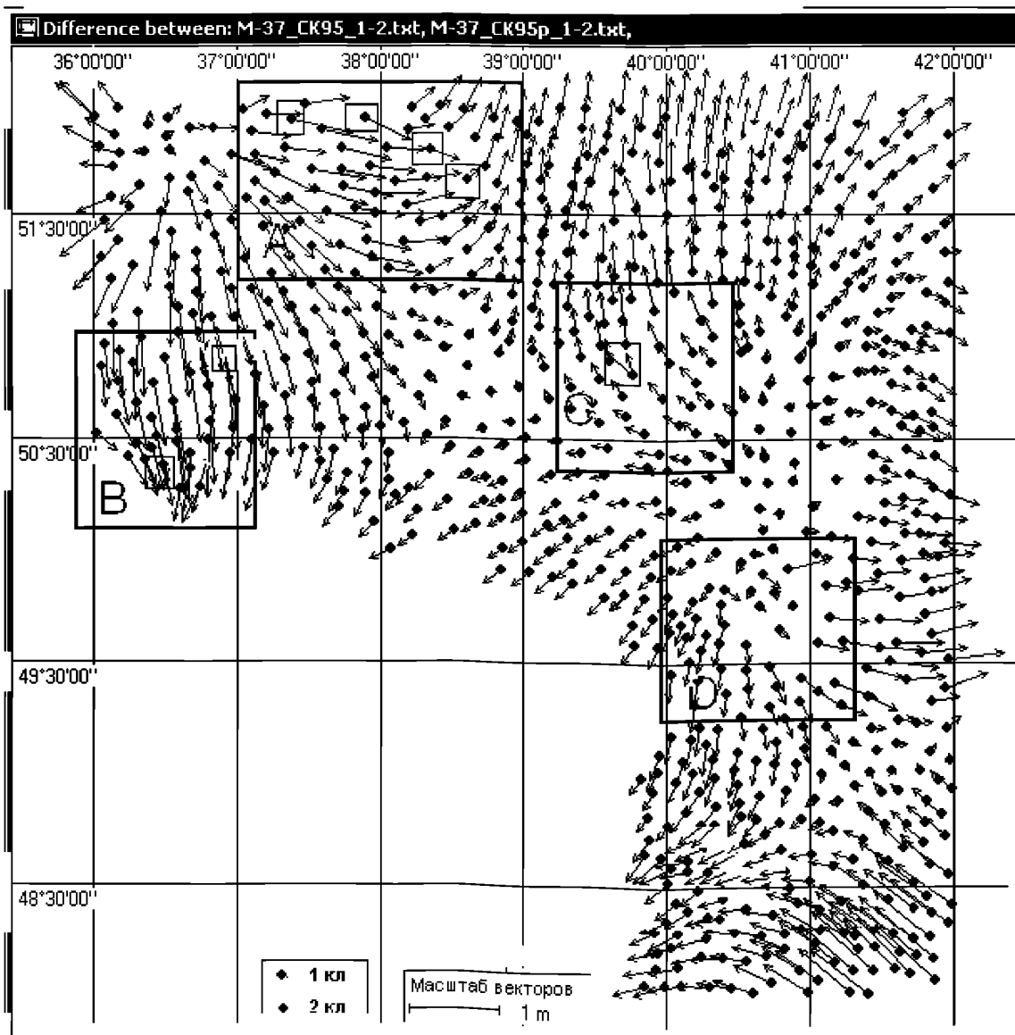
Рис. П6.1. Деформации СК42 на участке листа карты М37 м-ба 1:1000000
