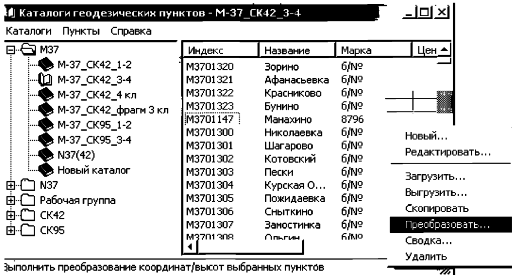
Рис. ПЗ.15 Вид окон при выполнении координатного преобразования на выбранной территории в библиотеке каталогов
