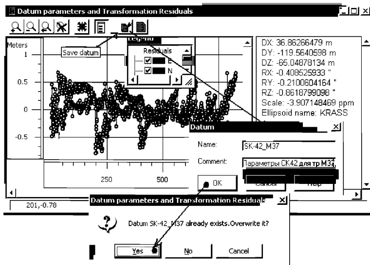
Рис. П5.10 Вид окна с результатами расчета параметров и графики величин остаточных невязок в плановых координатах пунктов
