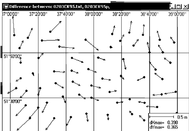
Рис. П6.3б. Остаточные расхождения координат на тр. М3702 и М3703
