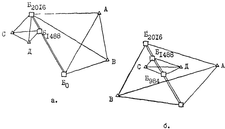
Рис.1 Схема расположения пунктов образцового базиса
