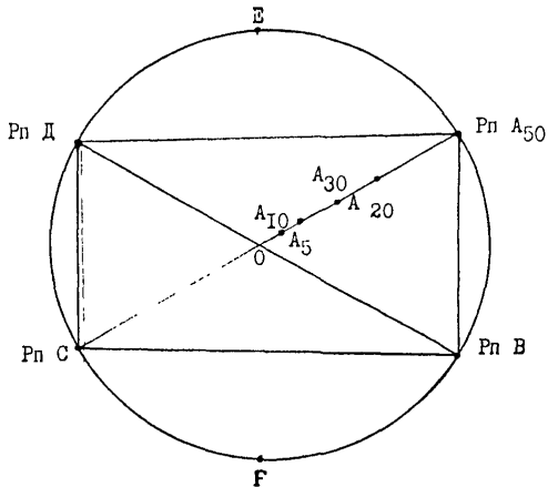
Рис.4 Схема контрольно-поверочной сети
