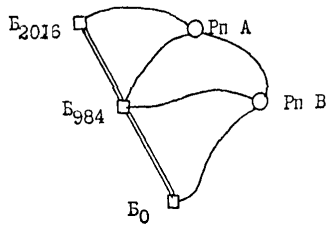
Рис.3 Схема нивелирного полигона
