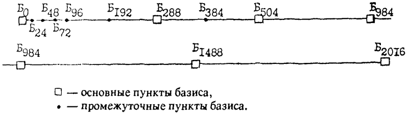
Рис.1 Схема расположения пунктов образцового базиса
