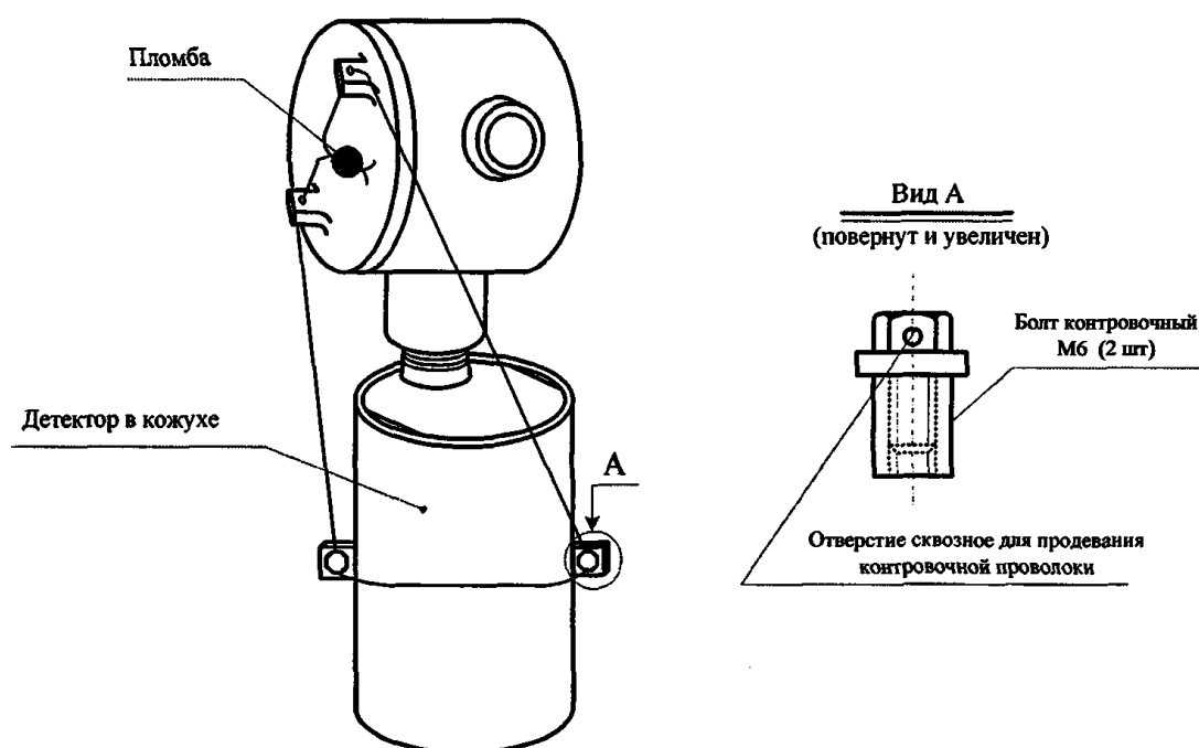
Рисунок Ж.6 – Пломбирование детектора модели В-5 фирмы «Smith Meter Inc.»
