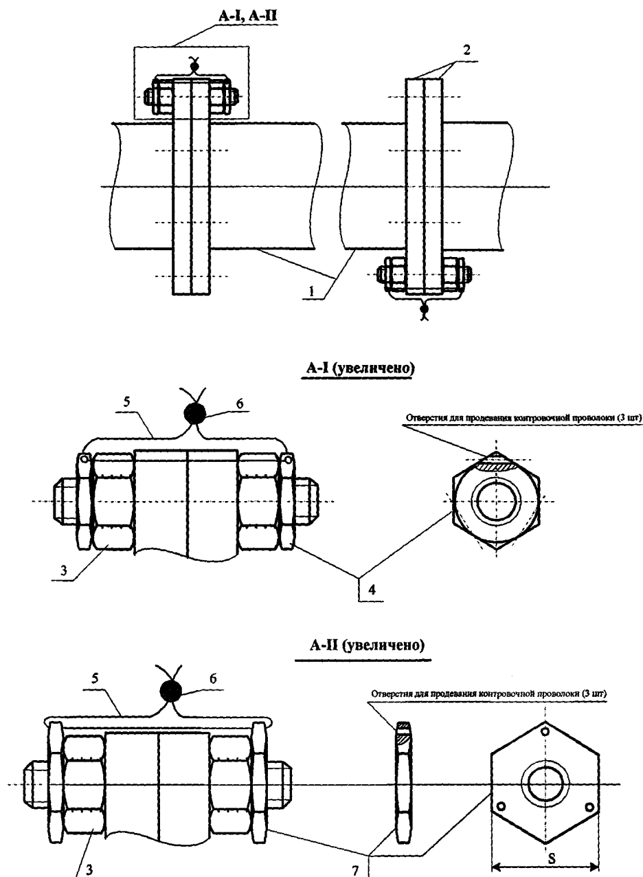
Рисунок Ж.1 – Пломбирование калиброванного участка ТПУ
