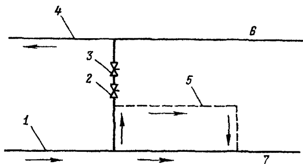
Рис. 3.2. Принципиальная схема прогрева отключенного участка байпаса промцерегрева (при плотной арматуре байпаса):
