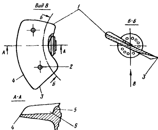
Рис. 3.15. Схема лопасти рабочего колеса поворотно-лопастной гидротурбины с указанием основных мест контроля:
