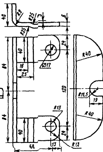
Рис. 2.3 Ограничитель хода золотника
