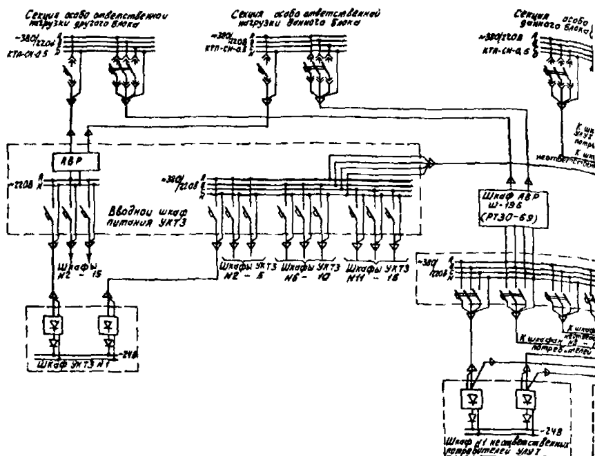
Рис. 4.2. Схема электропитания
