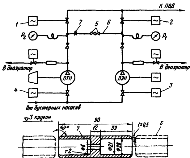
Рис. 2.5. Схема проверки плотности обратных клапанов питательных насосов:
