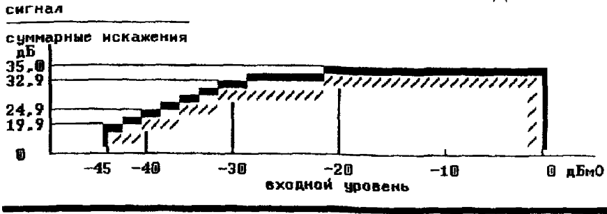
Рисунок 4 8 - Пределы суммарных искажений на входе соединения при L_1 = 0 дБ интерфейса Z
