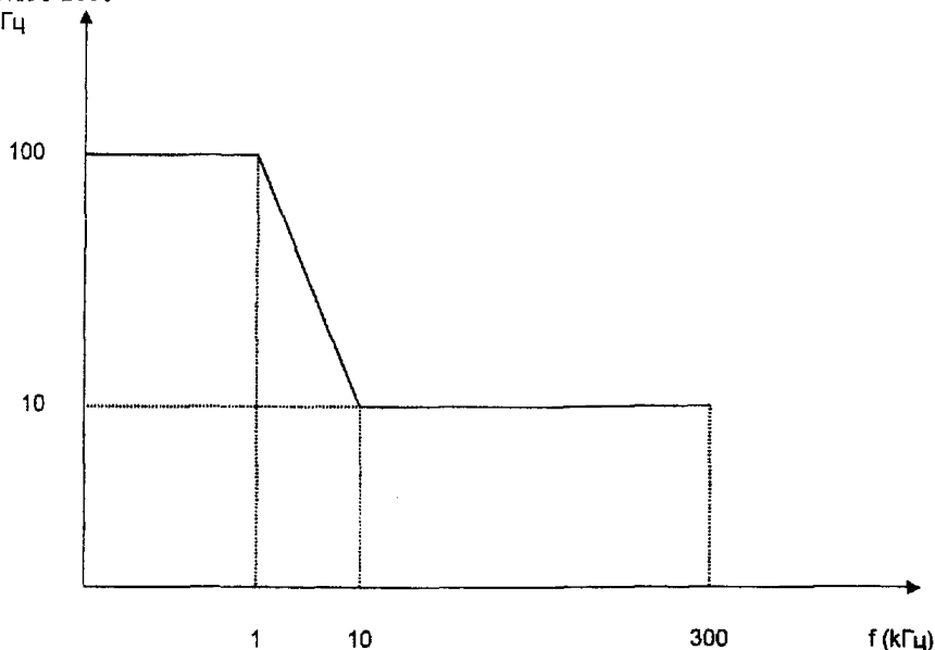
Рисунок П.2 - Импульсный шум
