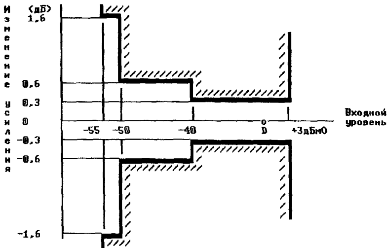
Рисунок 4 4 - Амплитудная характеристика на входе/выходе соединения (полусоединений)
