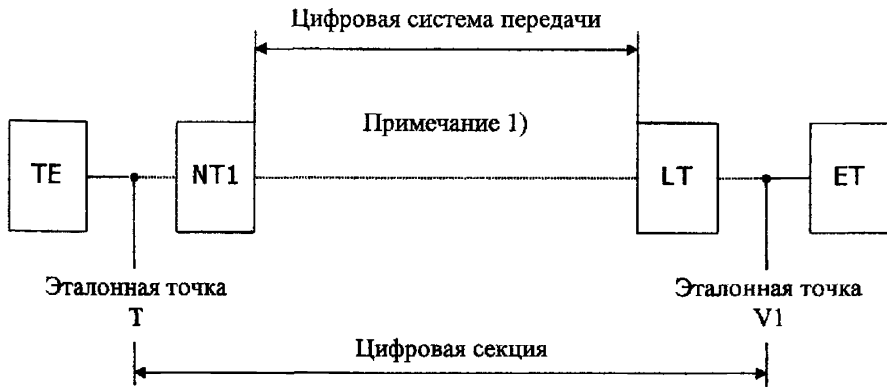
Рисунок П.1 – Цифровая секция
