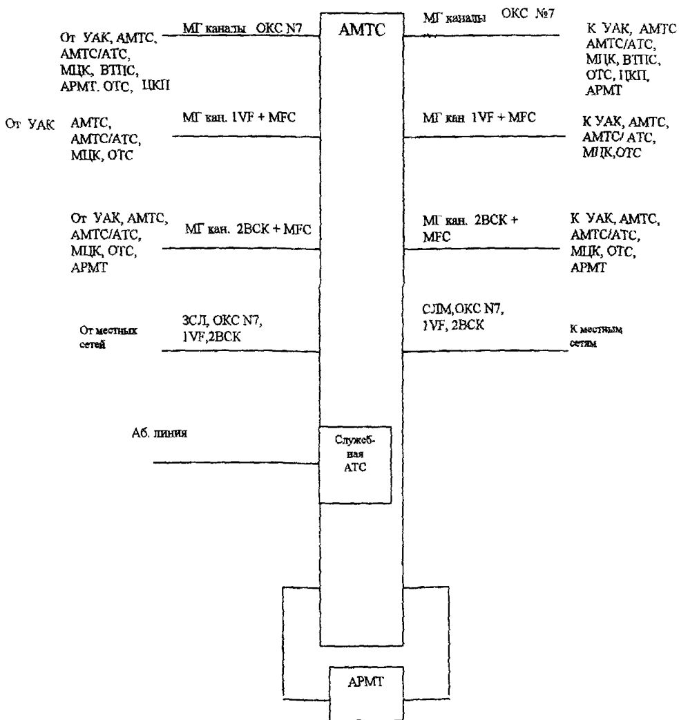
Рисунок 4.1 - Каналы и линии, включаемые в АМТС
