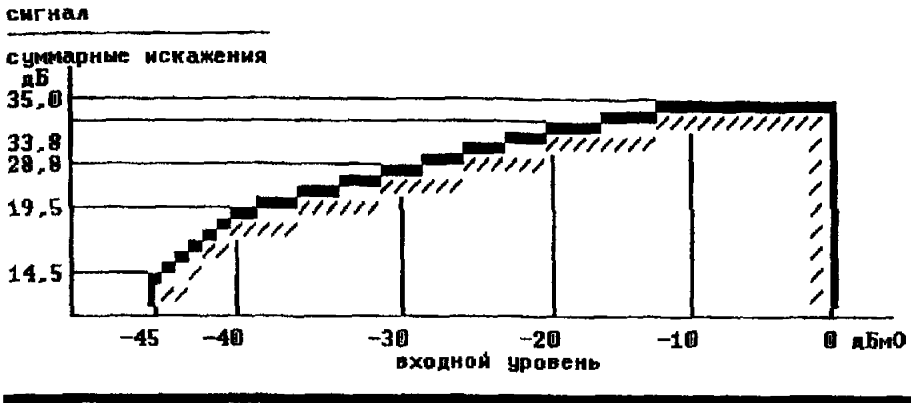
Рисунок 4 8 - Пределы суммарных искажений на входе соединения при L_1 = 0 дБ интерфейса Z
