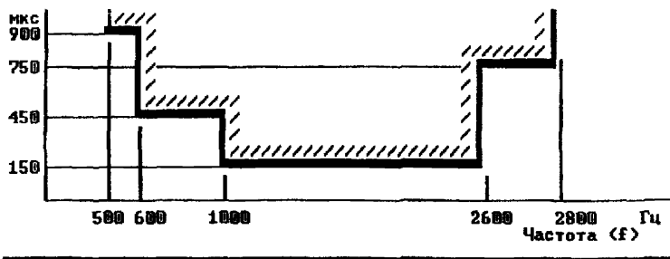
Рисунок 4.5 - Пределы отклонения группового времени прохождения между интерфейсами Z, A и A-Z
