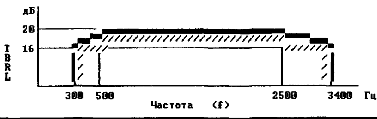
Рисунок 4.10 - Пределы балансного затухания дифсистемы
