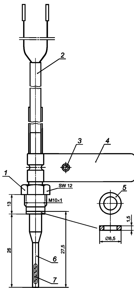
1 — зажимная гайка; 2 — соединительный кабель; 3 — место для опломбирования (пример); 4 — идентификационная пластина (пример); 5 — уплотнительное кольцо (материал: например, Си или РТФЕ); 6 — защитный корпус датчика температуры; 7 — термочувствительный элемент
