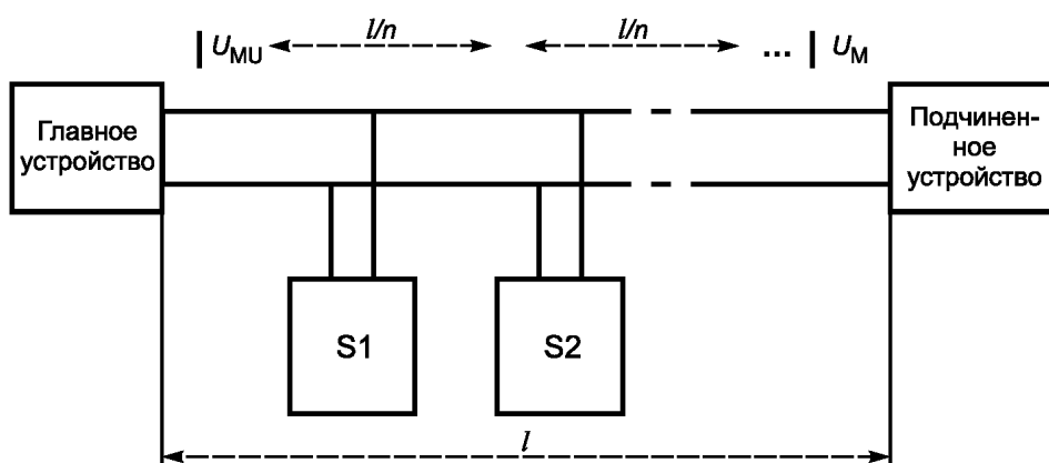
Рисунок В.3 — Тестовое оборудование для M-Bus ( l )
