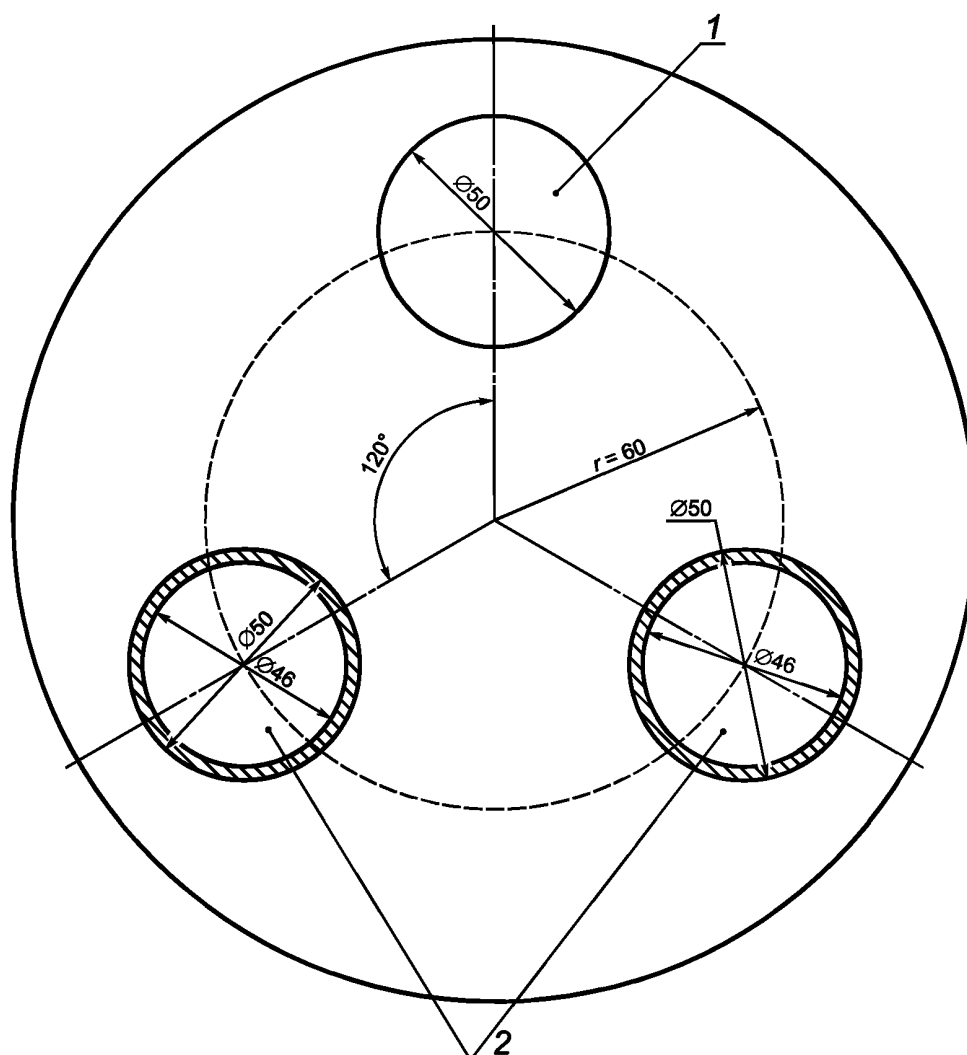
1 — твердый политетрафлюорэтилен; 2 — наполненные цилиндры
