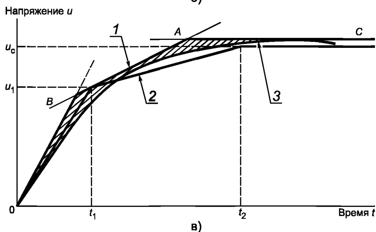
Рисунок 8 — Построение огибающей ПВН, определяемого четырьмя параметрами
