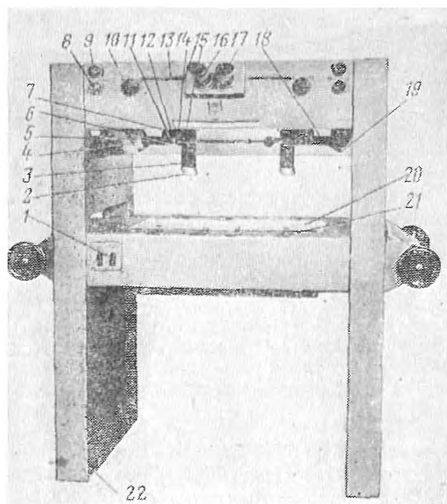
Рис. 7.1. Интерпретоскоп
