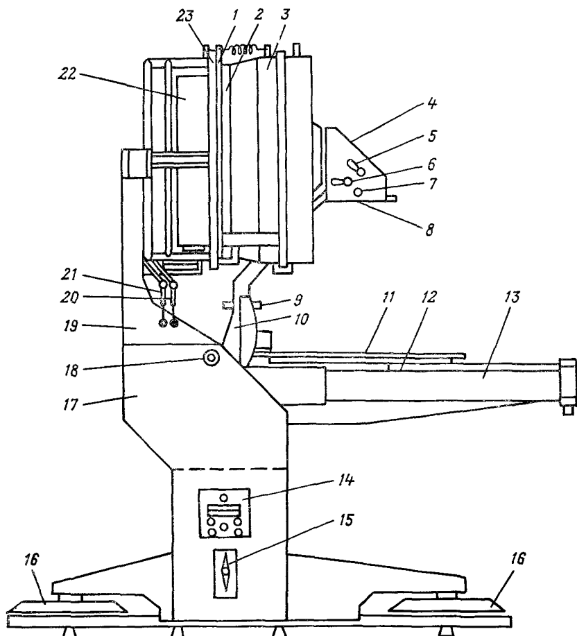
Рис. 6.2. Схема прибора
