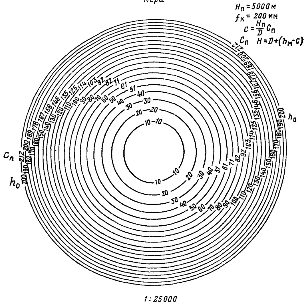
Рис 32 Палетка для определения поправок в показания радиовысотомера
