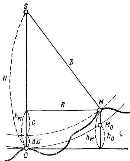
Рис 31. Определение высоты фотографирования
