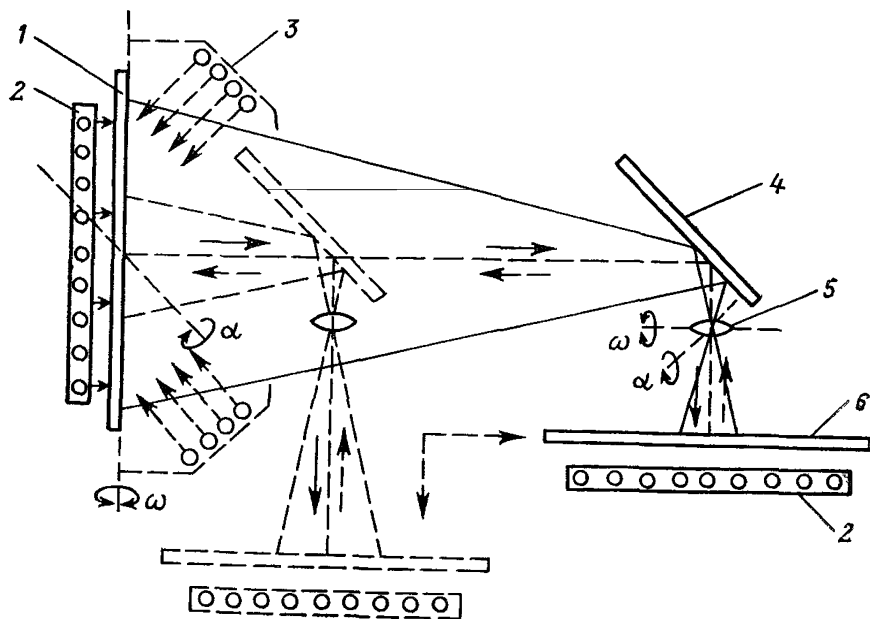
Рис. 6.1. Принцип проектирования
