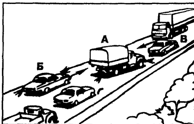
Рис.37. Обгон «вслед».
