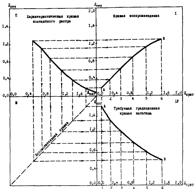
Рис. I. Определение требуемой градационной кривой полутонного негатива
