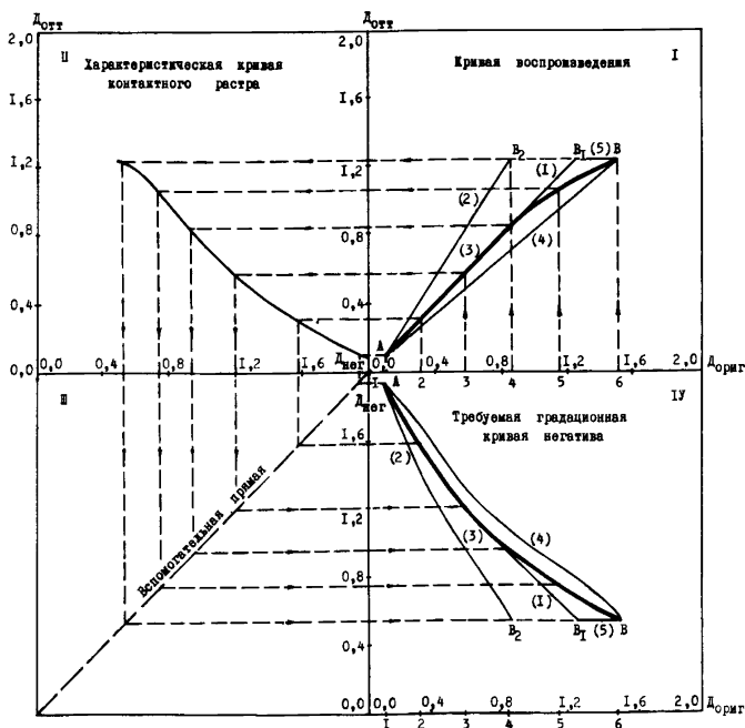
Рис.5. Определение требуемой градационной кривой цветоделенных полутоновых негативов
