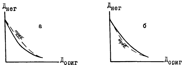
Рис.4. Неправильное экспонирование: а - недодержка, б - передержка
