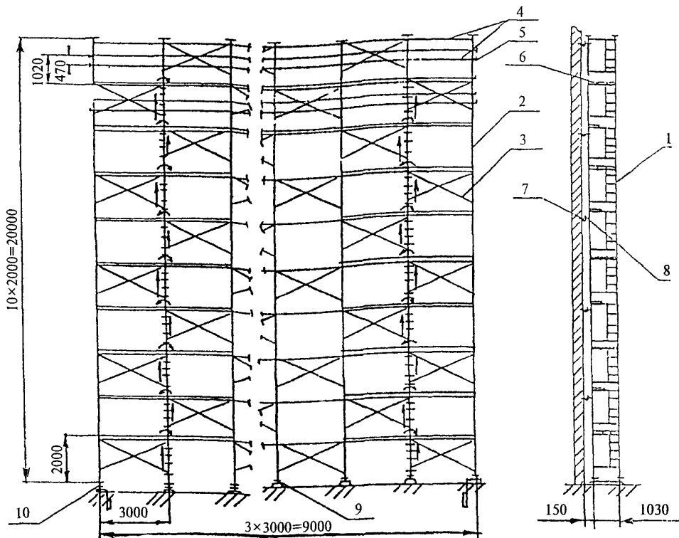
1 — рама с лестницей; 2 — рама; 3 — стяжка диагональная; 4 и 5 — стяжки ограждений; 6 — настил; 7 — пробка (или крюк со втулкой); 8 — стяжка; 9 — опора; 10 — опора винтовая
