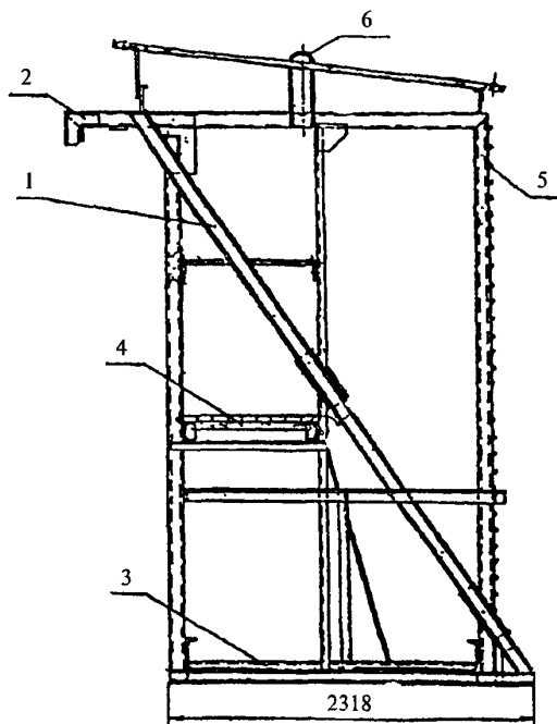
1 — рама; 2 — опора; 3 — настил; 4 — щит; 5 — сетка; 6 — петля
