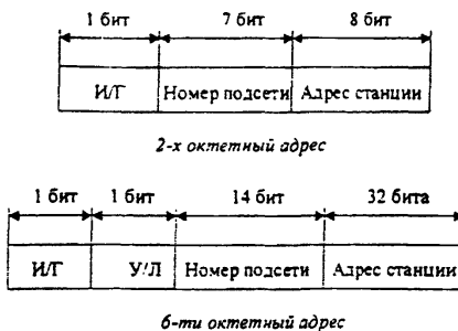
Рисунок 6.3 – Формат полей АП и АО
