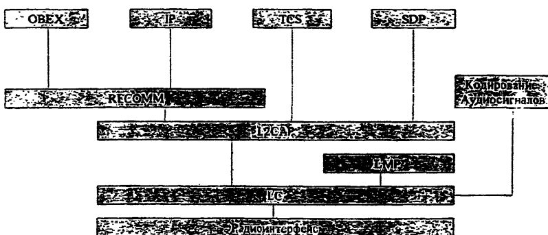
Рисунок 6.8 – Протоколы и функции, реализуемые аппаратурой Bluetooth
